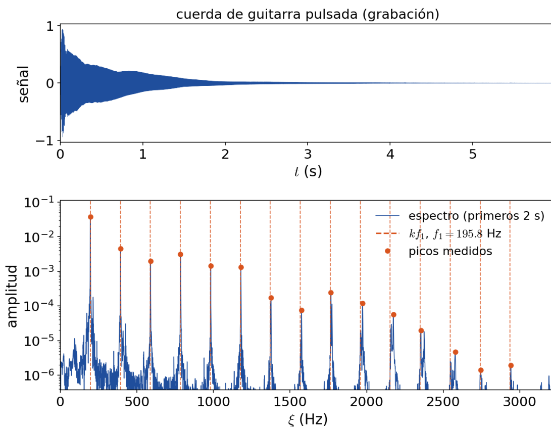
FIGURA 17.2. Grabación de una cuerda de guitarra pulsada (la tercera cuerda, Sol) y su espectro de amplitudes calculado con los primeros dos segundos. Las líneas de trazos marcan los múltiplos kf_1 de la fundamental medida, f_1 = 195,8 Hz: los picos están casi exactamente allí, pero el desvío crece con k (inarmónica) y las amplitudes de los armónicos altos son mucho menores. Los datos están en el repositorio de la materia (datos/cuerda_guitarra.wav).
