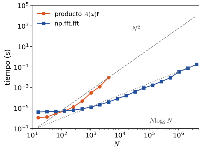
FIGURA 14.5. Tiempo de cómputo de la DFT por producto con la matriz A(\omega) y con la FFT ( np.fft.fft ) en función de N , con las referencias N^2 y N \log_2 N . Para N = 4096 la FFT es unas 300 veces más rápida.
