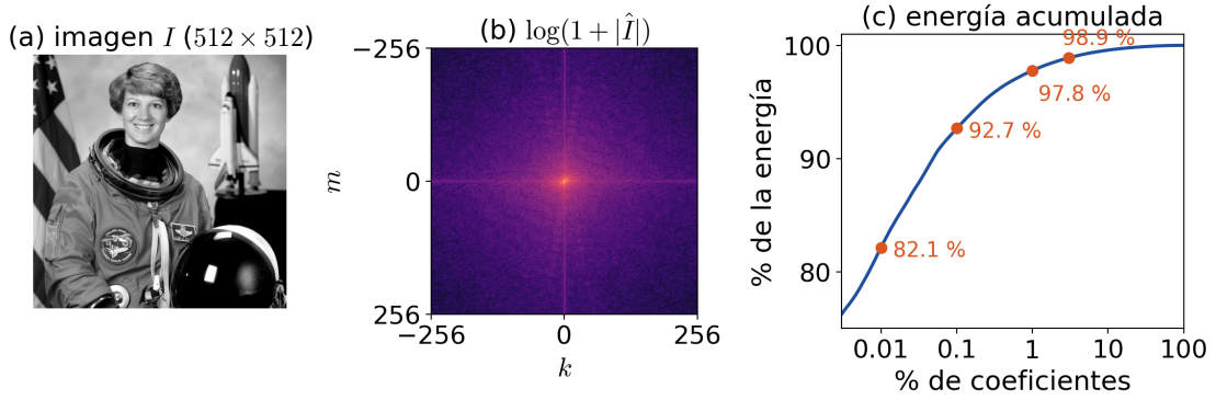
FIGURA 15.7. (a) La imagen (fotografía de la astronauta Eileen Collins, NASA, dominio público, distribuida con scikit-image ). (b) \log(1 + |\hat{I}|) con el origen de frecuencias en el centro: la energía se concentra en las bajas frecuencias. (c) Fracción de la energía \sum |\hat{I}|^2 contenida en los coeficientes de mayor módulo: el 1 % tiene el 97,8 % y el 0,1 % el 92,7 %.
