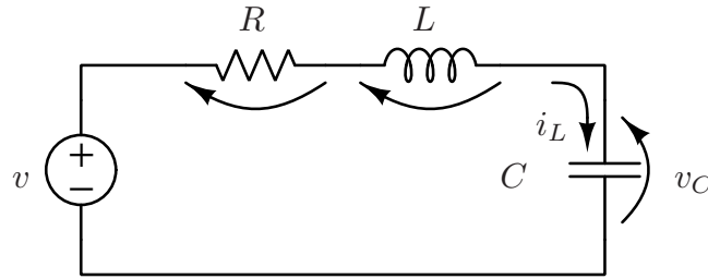
FIGURA 9.1. Circuito RLC serie (Ejercicio 9.2.20).
