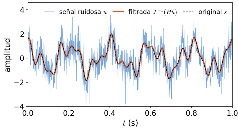
FIGURA 15.4. Señal filtrada
