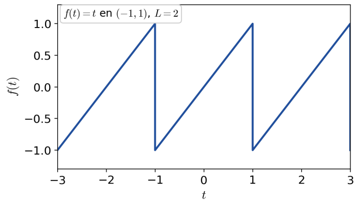
FIGURA 12.9. Función diente de sierra.
