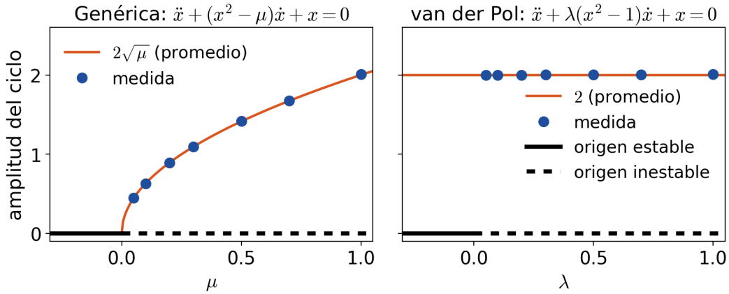
FIGURA 8.13. Hopf genérica frente al caso degenerado, con la amplitud del ciclo medida numéricamente. Izquierda: la familia \ddot{x} + (x^2 - \mu)\dot{x} + x = 0 , cuyo ciclo nace en \mu = 0 con amplitud 2\sqrt{\mu} . Derecha: van der Pol, donde el ciclo aparece con amplitud \approx 2 para todo \lambda > 0 .
