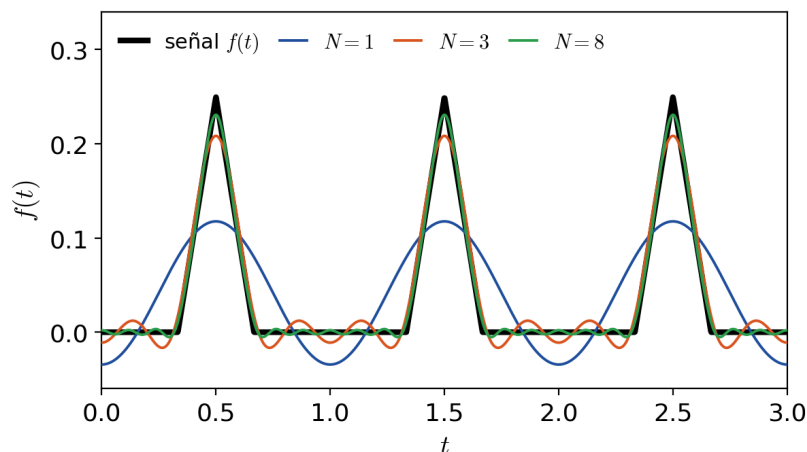
FIGURA 11.3. Aproximación de la señal superponiendo 1, 3 y 8 frecuencias.
