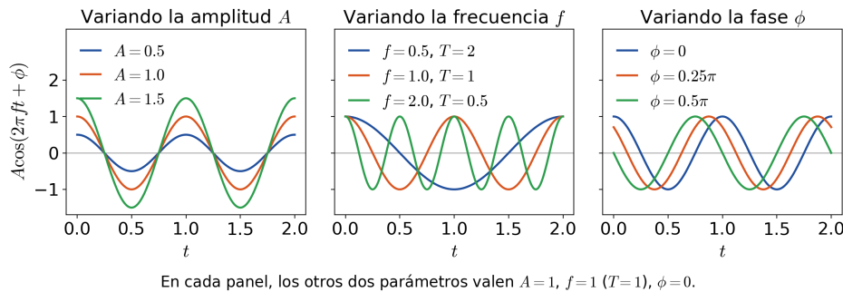
FIGURA 11.1. Ondas fundamentales con distintas amplitudes, frecuencias y fases.
