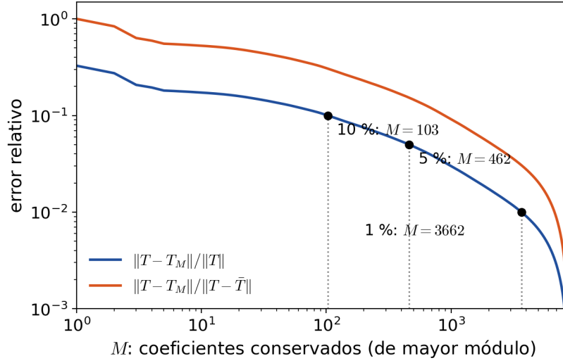
FIGURA 15.6. Error relativo de la reconstrucción de la serie de temperatura de 2023 conservando los M coeficientes de mayor módulo (calculado con Plancherel), respecto de \|T\| y de \|T - \bar{T}\| . Para un 10 % alcanzan 103 coeficientes, para un 5 % hacen falta 462 y para un 1 %, 3662 de 8760.
