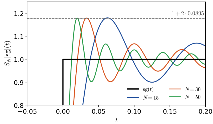
FIGURA 12.8. Detalle del fenómeno de Gibbs para la función signo.
