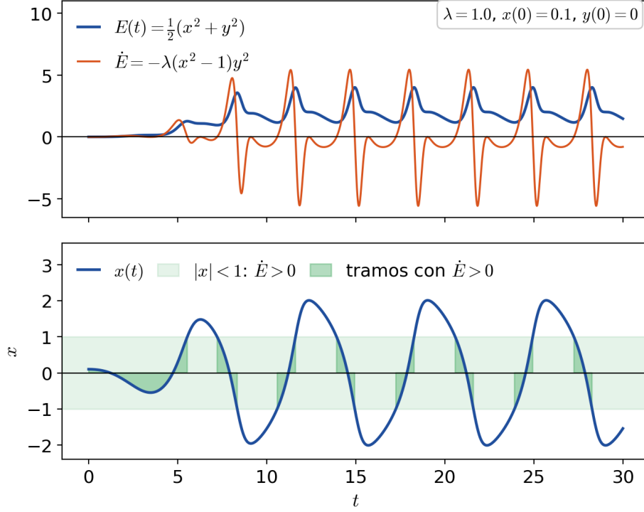
FIGURA 3.3. La “energía” E = \frac{1}{2}(x^2 + y^2) a lo largo de una solución de van der Pol ( \lambda = 1, x(0) = 0.1, y(0) = 0 ): \dot{E} = -\lambda(x^2 - 1)y^2 es positiva mientras |x| < 1 y negativa cuando |x| > 1 , así que E no es monótona. La solución termina oscilando con E entre 1,17 y 4; la amplitud de esa oscilación no depende de la condición inicial.
