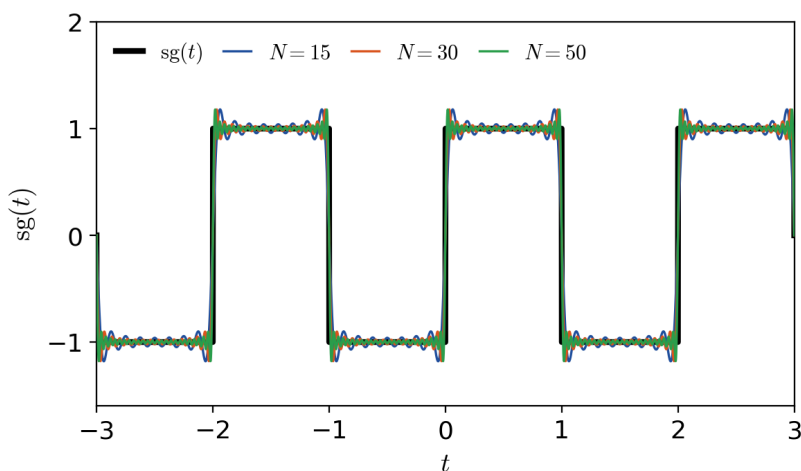
FIGURA 12.7. Fenómeno de Gibbs para la función signo.
