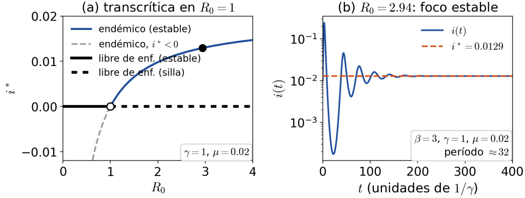
FIGURA 8.14. SIR con nacimientos (8.6.1), \gamma = 1 , \mu = 0,02 . (a) Diagrama de bifurcación: la rama endémica i^* = \frac{\mu}{\beta}(R_0 - 1) intercambia estabilidad con la libre de enfermedad en R_0 = 1 ; el punto lleno es el equilibrio del panel (b). (b) Con \beta = 3 ( R_0 \approx 2,94 ) el equilibrio endémico es un foco estable: i(t) se acerca a i^* con ondas de período \approx 32 (escala logarítmica).
