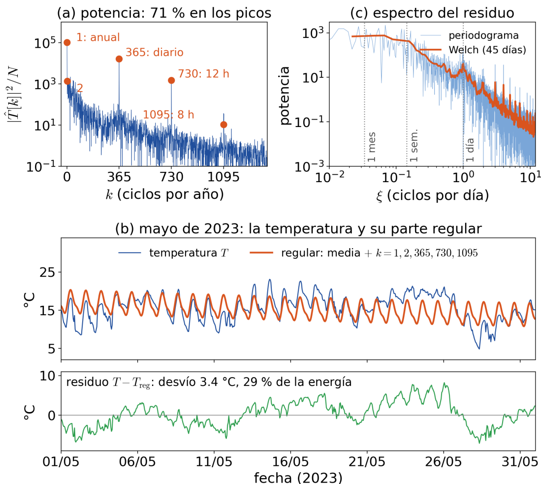
FIGURA 15.5. La temperatura horaria de 2023 y sus ciclos. (a) Espectro de potencia |\hat{T}[k]|^2/N con los picos anual ( k = 1 ), semestral ( k = 2 ), diario ( k = 365 ) y sus armónicos (730, 1095): entre los cinco contienen el 71 % de la energía fuera de la media. (b) Un mes de la señal y la “temperatura regular” (media más los cinco picos) obtenida filtrando; debajo, el residuo irregular (desvío 3,4 °C, 29 % de la energía). (c) Espectro del residuo en ciclos por día (periodograma y promedio de Welch): no es blanco, decae como \xi^{-1,7} y tiene la mayor parte de su energía en períodos de días a semanas (frentes).
