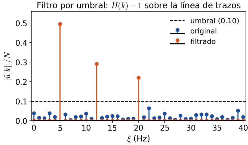
FIGURA 15.3. Filtro usado
