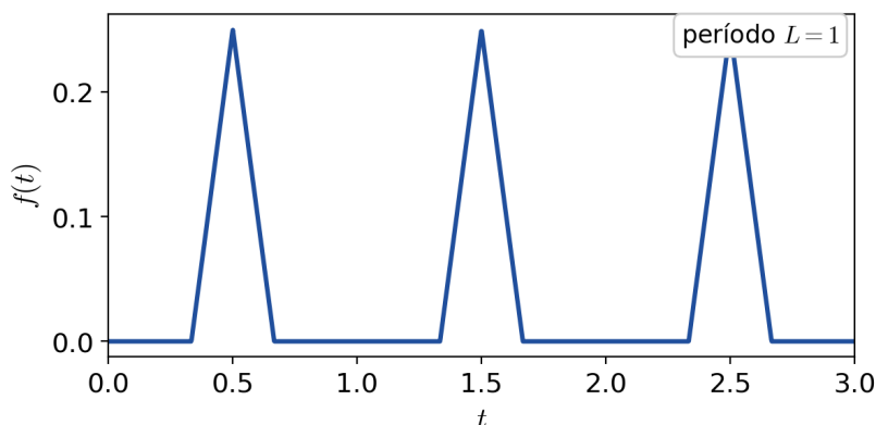
FIGURA 11.2. Ejemplo de señal periódica.
