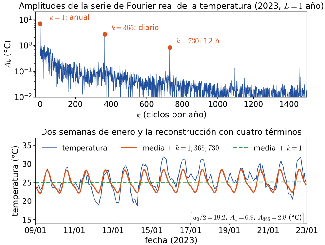
FIGURA 11.4. Serie de Fourier real de la temperatura de 2023 ( L = 1 año). Arriba: amplitudes A_k ; sobresalen el ciclo anual ( k = 1 , A_1 \approx 6,9 °C), el diario ( k = 365 , A_{365} \approx 2,8 °C) y su primer armónico ( k = 730 ). Abajo: dos semanas de enero y la reconstrucción con sólo la media y esos tres términos, que explican el 70 % de la varianza.
