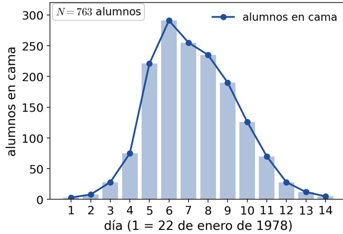
FIGURA 1.1. Alumnos en cama por día durante la epidemia de gripe en un internado inglés de 763 alumnos, del 22 de enero al 4 de febrero de 1978 [1]. Es el dato que se ajusta en el laboratorio de la Parte I.
