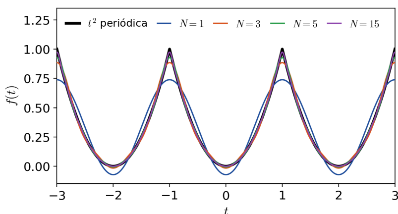
FIGURA 12.5. Aproximaciones de f(t) = t^2 mediante Fourier.
