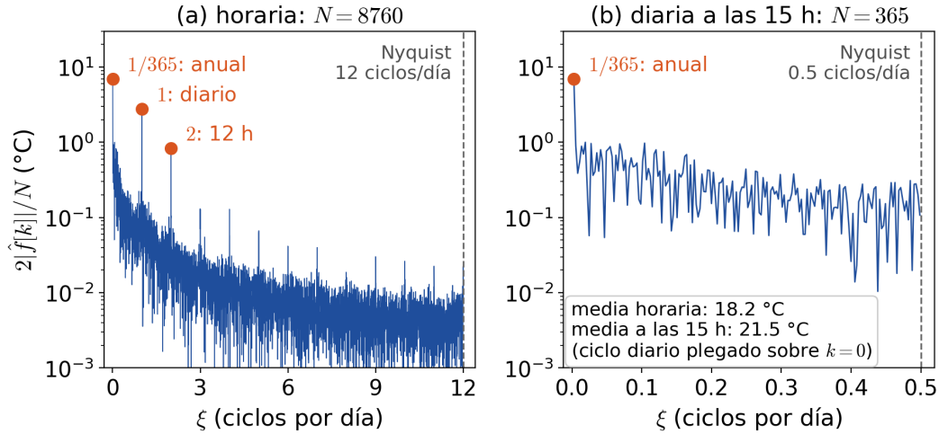
FIGURA 14.3. (a) Espectro de amplitudes de la temperatura horaria de 2023 en ciclos por día, hasta la frecuencia de Nyquist (12 ciclos/día); se marcan el ciclo anual ( 1/365 ), el diario (1) y su armónico de 12 h (2). (b) Espectro de la misma señal muestreada una vez por día a las 15 h: la frecuencia de Nyquist baja a 0,5 ciclos/día, el ciclo anual sigue intacto y el diario se pliega sobre k = 0 : la media sube de 18,2 a 21,5 °C.
