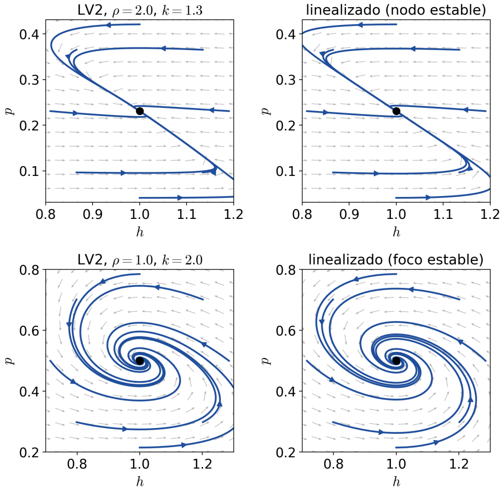
FIGURA 5.9. Hartman–Grobman en el modelo (2.3.2): a la izquierda el sistema en una ventana alrededor del equilibrio de coexistencia (1, 1 - 1/k) , a la derecha el sistema linealizado \dot{\mathbf{y}} = DF(\mathbf{x}^*)\mathbf{y} en las mismas coordenadas y con las mismas condiciones iniciales. Arriba \rho^2 \geq 4k(k-1) (nodo estable), abajo \rho^2 < 4k(k-1) (foco estable).
