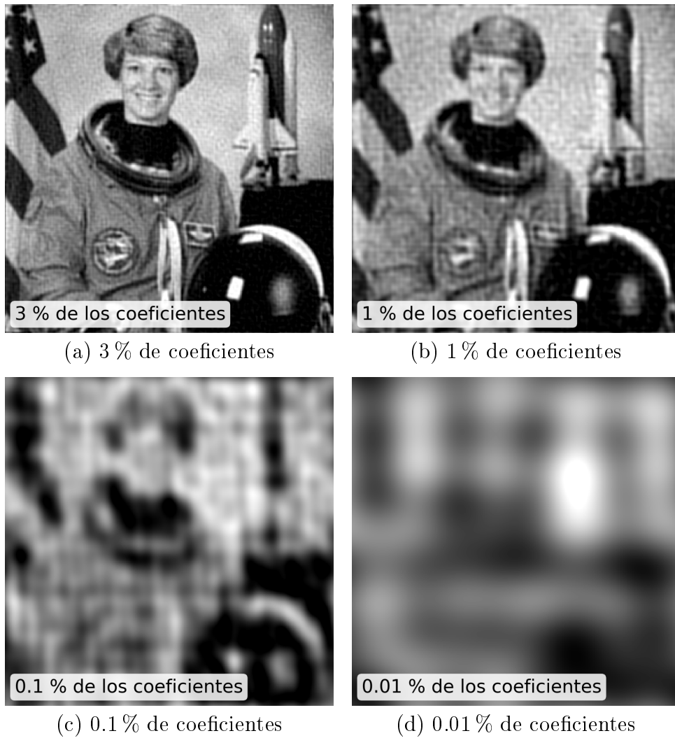
FIGURA 15.9. Reconstrucción de la imagen mediante truncamiento espectral, conservando distintos porcentajes de los coeficientes de Fourier de mayor magnitud. Error relativo en norma 2: 0,11 (3 %), 0,15 (1 %), 0,27 (0,1 %), 0,42 (0,01 %).
