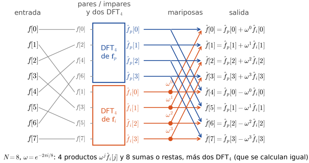
FIGURA 14.4. Una etapa del algoritmo de Cooley–Tukey para N = 8 : se separan las coordenadas pares e impares, se calculan dos DFT de tamaño 4 y se combinan de a pares (“mariposas”) con los factores \omega^j , \omega = e^{-2\pi i/8} : \hat{f}[j] = \hat{f}_p[j] + \omega^j \hat{f}_i[j] , \hat{f}[j + 4] = \hat{f}_p[j] - \omega^j \hat{f}_i[j] .
