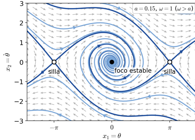
FIGURA 5.7. Diagrama de fases para (5.3.1).
