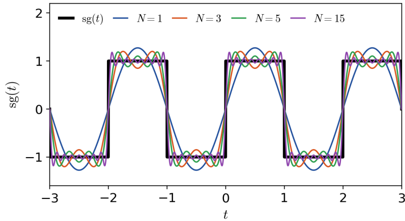
FIGURA 12.3. Función signo y algunas aproximaciones usando la serie de Fourier.
