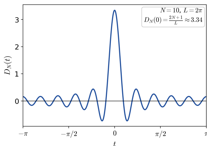
FIGURA 12.1. Núcleo de Dirichlet para N = 10 y L = 2\pi ; D_N(0) = (2N + 1)/L .
