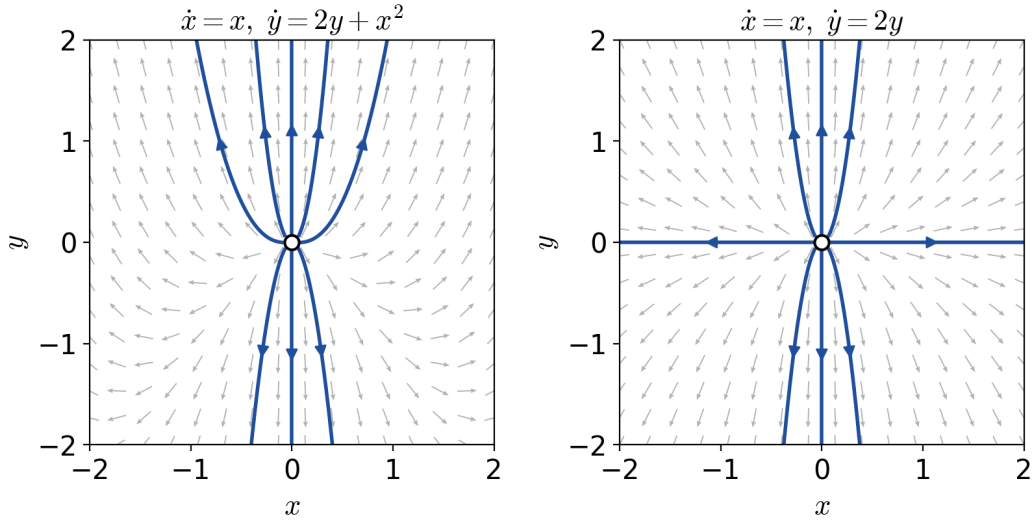
FIGURA 5.6. Los sistemas \dot{x} = x, \dot{y} = 2y + x^2 (izquierda) y su linealización \dot{x} = x, \dot{y} = 2y (derecha), con las mismas condiciones iniciales. Cerca del origen ambos son nodos inestables y el homeomorfismo \mathbf{h}(x, y) = (x, y - x^2 \ln |x|) lleva las trayectorias de uno en las del otro, pero ningún cambio de coordenadas de clase C^2 puede hacerlo.
