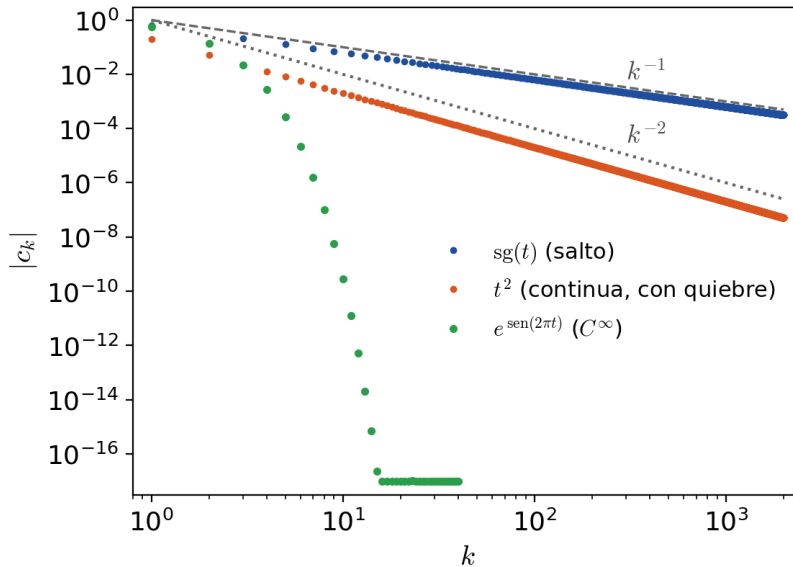
FIGURA 12.6. Decaimiento de los coeficientes de Fourier según la regularidad de la señal: la función signo (salto) decae como 1/k , t^2 extendida periódicamente (continua con un quiebre) como 1/k^2 y e^{\sin(2\pi t)} ( C^\infty ) más rápido que cualquier potencia.
