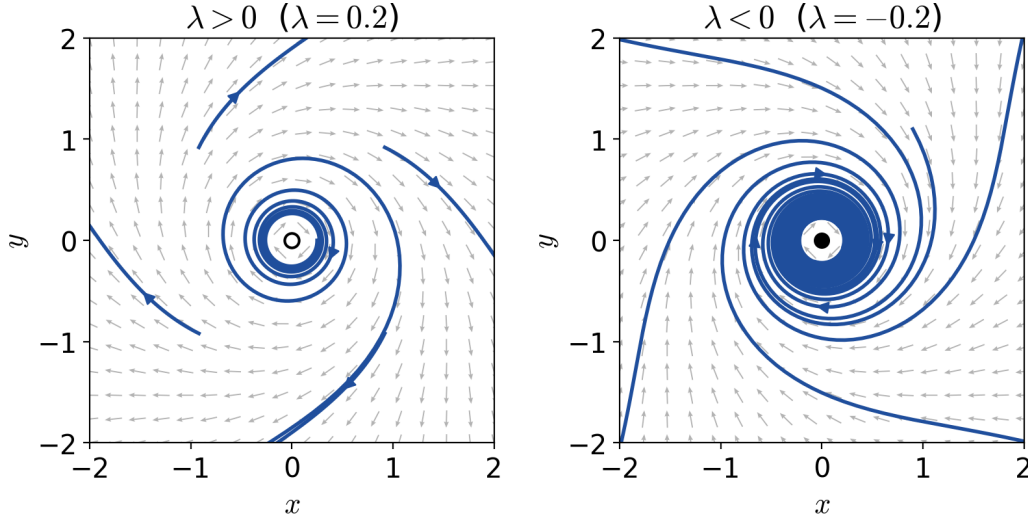
FIGURA 5.8. Diagrama de fases para (5.3.2). A la izquierda para \lambda > 0 y a la derecha para \lambda < 0 .
