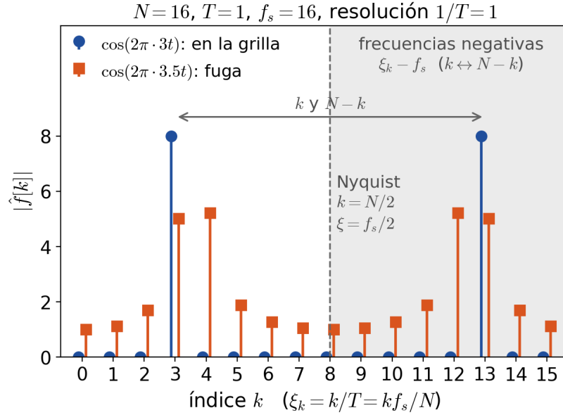
FIGURA 14.2. Grilla de frecuencias de la DFT con N = 16, T = 1 ( f_s = 16 ). |\hat{f}[k]| para \cos(2\pi \cdot 3t) , cuya frecuencia cae en la grilla (dos picos, k = 3 y N - k = 13 ), y para \cos(2\pi \cdot 3.5t) , que cae entre dos puntos y reparte su energía en todos los índices (fuga espectral). Los índices k > N/2 son las frecuencias negativas \xi_k - f_s ; la línea punteada es la frecuencia de Nyquist.
