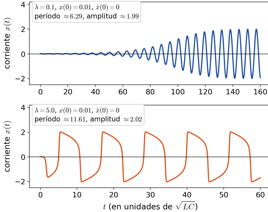
FIGURA 1.2. Corriente en el circuito de van der Pol (simulación) a partir de una perturbación pequeña del reposo. Arriba, \lambda = 0,1 : la corriente crece lentamente y se estabiliza en una oscilación casi sinusoidal de amplitud \approx 2 y período \approx 2\pi . Abajo, \lambda = 5 : el circuito se enciende de inmediato y oscila con forma de relajación, con período mucho mayor que el natural. En el laboratorio se trabaja con un registro de este tipo, con ruido.
