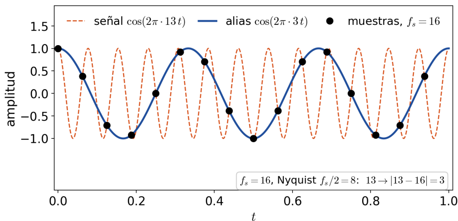
FIGURA 14.1. Ejemplo de aliasing: dos señales continuas con distintas frecuencias producen las mismas muestras discretas cuando la tasa de muestreo es insuficiente.
