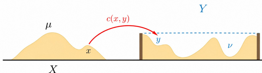
FIGURA P.1. El problema original de Monge: transportar una distribución de masa \mu sobre X hacia otra distribución \nu sobre Y , minimizando el costo total de transporte.
