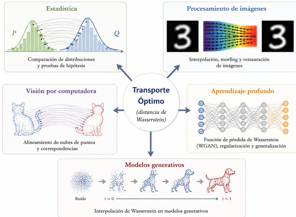
FIGURA P.3. Algunas aplicaciones contemporáneas del transporte óptimo y de la distancia de Wasserstein.
