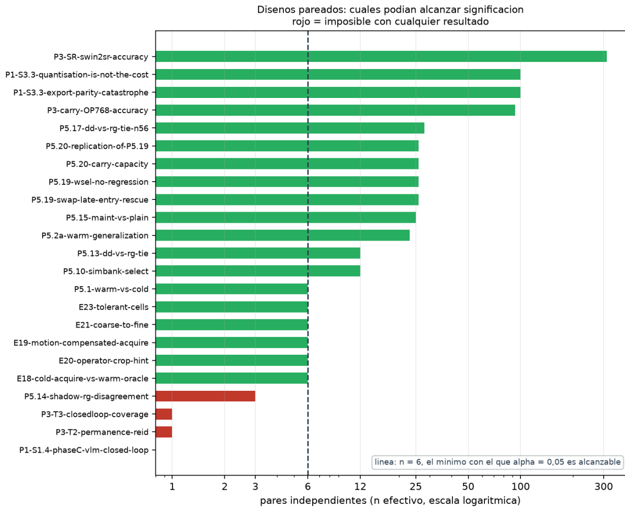
Figura 4.1: Diseños pareados por n efectivo; en rojo los que no podian alcanzar significacion con ningun resultado
