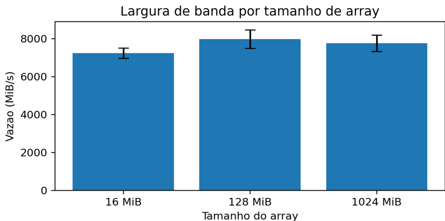
Figura 1. Largura de banda da memória para diferentes tamanhos de array com IC 95%.
