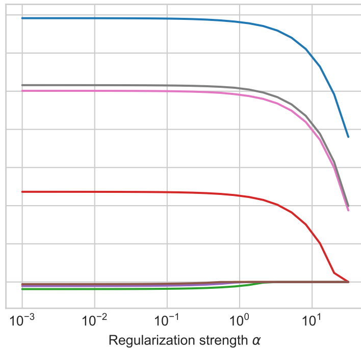
Lasso
