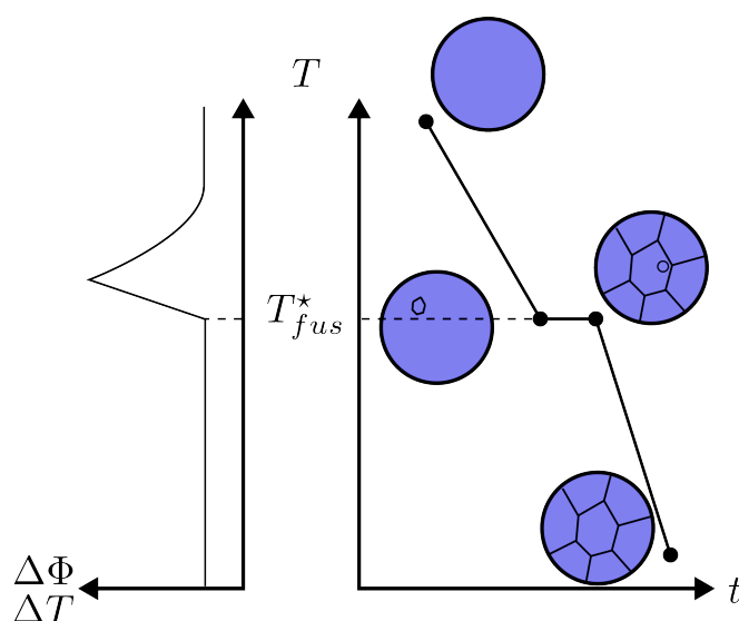
Figure 2.4 – Exemple théorique de la fusion ou solidification du corps pur A à l'aide de la DSC ou du refroidissement thermique.
