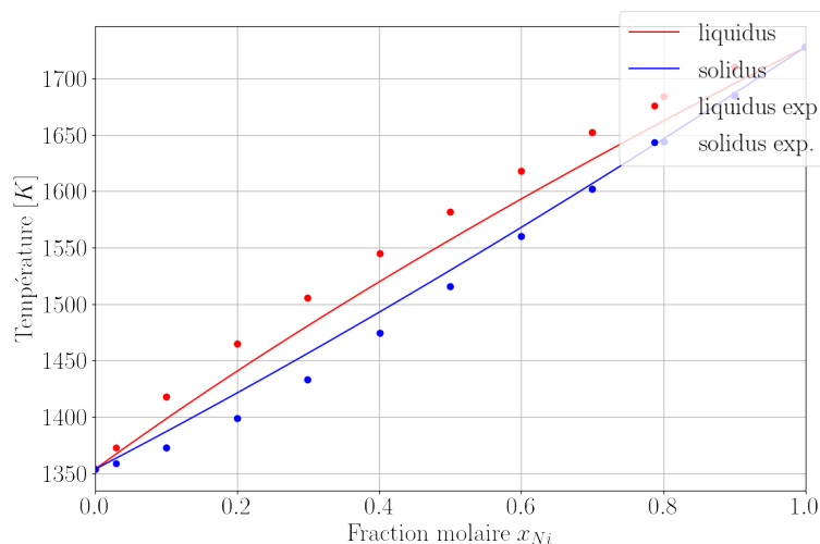
Figure 2.10 - Diagramme isobare Cu-Ni à une pression de 1 bar modélisée à l'aide de l'équation de Schröder-van Laar
