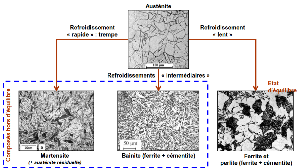
Figure 2.38 – Bilan : effet de la vitesse de refroidissement sur les transitions de phases de l'austénite
