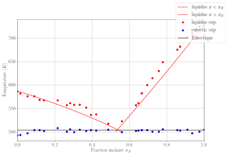
Figure 2.14 – Diagramme de phase d'un solide hétérogène AgCl-ZnCl 2 à miscibilité nulle, isobare, à une pression de 1 bar
