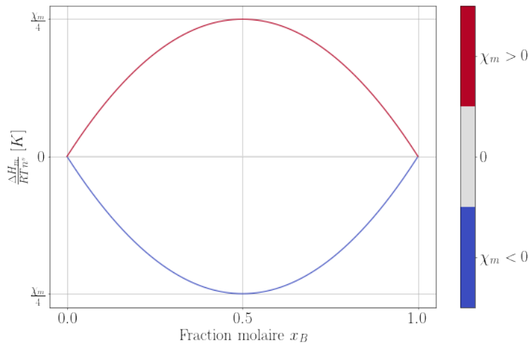
Figure 2.5 – Enthalpie de mélange dans le cas d'une interaction A–B défavorable \chi_m > 0 , d'une interaction A–B équivalente A–A et B–B \chi_m = 0 et d'une interaction A–B favorable \chi_m < 0
