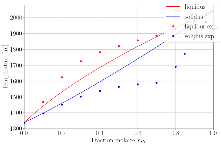
Figure 2.11 – Diagramme isobare Au-Pt à une pression de 1 bar modélisée à l’aide de l’équation de Schröder-van Laar
