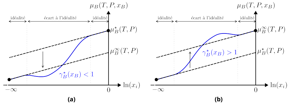
Figure 2.3 – Evolution du potentiel chimique d'un constituant B en fonction de la fraction molaire en échelle logarithmique dans le cas d'une interaction A–B plus favorable (2.3a) que les interactions A–A et B–B (2.3b) défavorable
