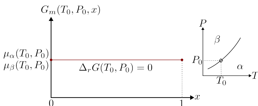
Figure 1.19 – Allure de G en fonction de la fraction x en phase \beta dans le cas où la phase \alpha est aussi stable que la phase \beta . Position correspondante dans le diagramme (P, T)
