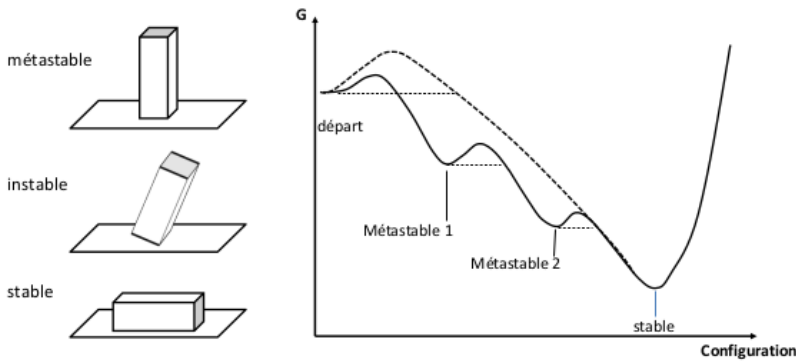
Figure 1.23 – Profil d'enthalpie libre présentant des minimums locaux (états métastables) et un minimum absolu (état d'équilibre)
