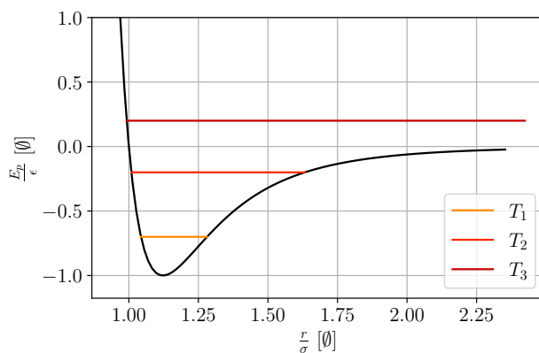
Figure 1.5 – Potentiel de Lennard-Jones, normalisé par les paramètres du modèle (\epsilon, \sigma)
