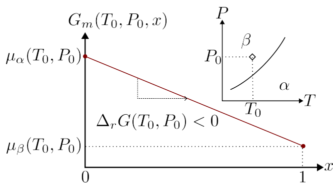
Figure 1.17 – Allure de G en fonction de la fraction x en phase \beta dans le cas où la phase \beta est la plus stable. Position correspondante dans le diagramme (P, T)
