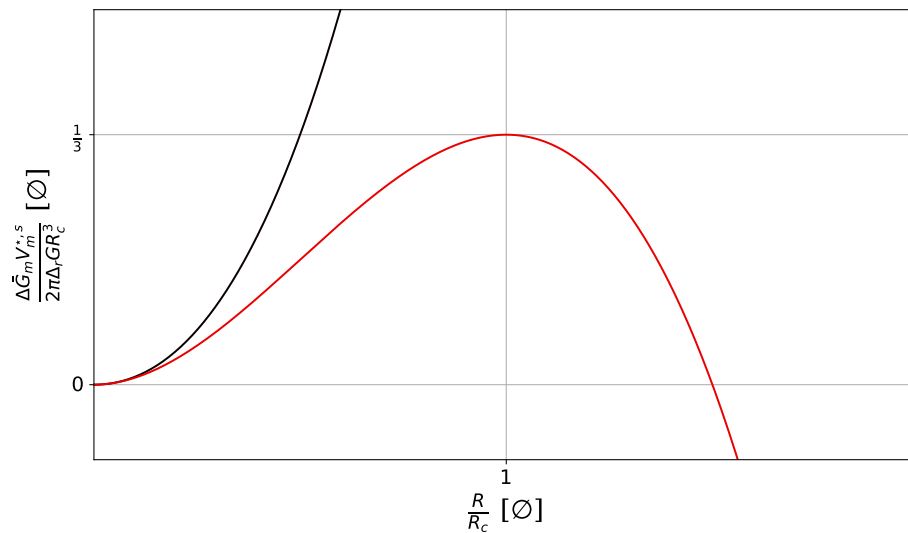
Figure 1.24 – Evolution d’une fonction normalisée de l’enthalpie libre en fonction du rayon du cristal.
