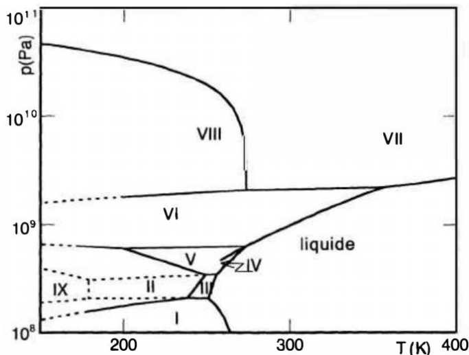
Figure 1.12 – Diagramme de phase pression-température, zoomé sur les hautes pressions ( P > 10^8 Pa), en échelle lin-log, représentant les domaines de stabilité, des différents polymorphes de l'eau solide.
