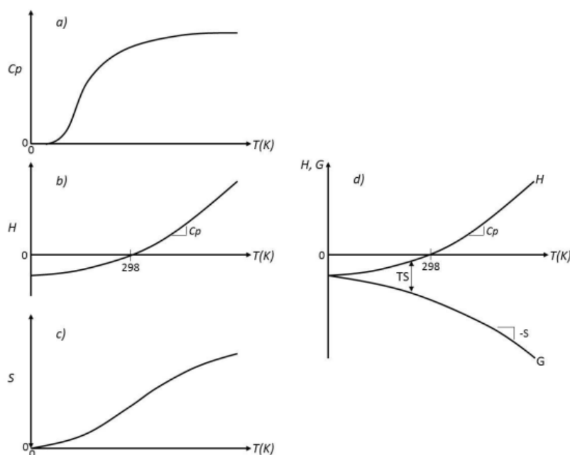
Figure 1.16 – Représentation de l'évolution de plusieurs grandeurs thermodynamiques avec la température lors de l'échauffement d'un solide à pression constante.
