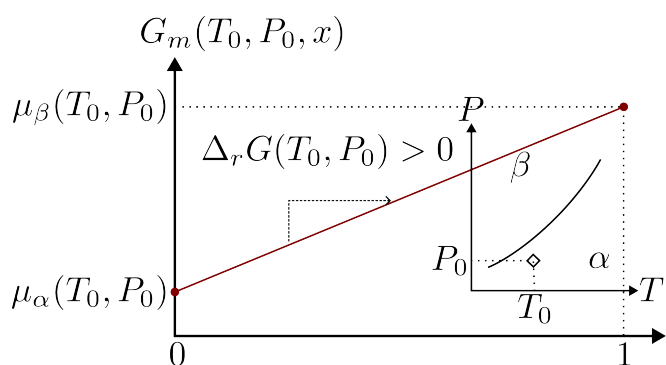
Figure 1.18 – Allure de G en fonction de la fraction x en phase \beta dans le cas où la phase \alpha est la plus stable. Position correspondante dans le diagramme (P, T)
