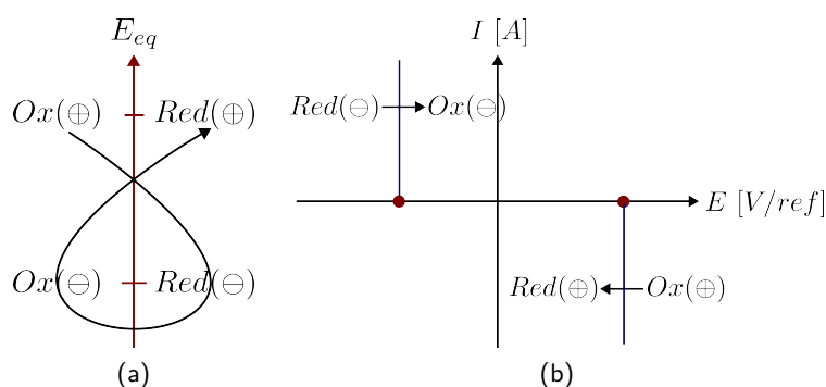
Figure 13 – 13a Axe de potentiel thermodynamique; 13b Courbe courant-potentiel dans le cas idéal où le transfert d'électron serait infiniment rapide, construite à partir de l'axe de potentiel thermodynamique en utilisant la convention I > 0 : oxydation, I < 0 : réduction
