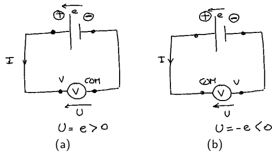
Figure 3 – 3a Circuit équivalent permettant d'obtenir une tension positive ; 3b Circuit équivalent permettant d'obtenir une tension négative.
