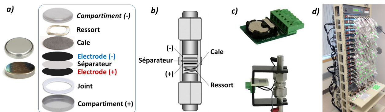
Figure 8 – Une demi-cellule électrochimique peut-être étudiée en utilisant une pile bouton (a), un cellule Swagelok©(b) et peuvent être installés sur un cycleur capable d'évaluer en parallèle les performances de cyclage de dizaines de batteries (c & d).
