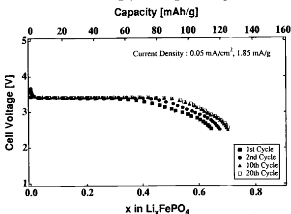
FIGURE 18 – Évolution du potentiel cathodique par rapport à une électrode au lithium pour une densité de courant de 0.05 mA en fonction de la fraction en lithium dans \text{Li}_x\text{FePO}_4 .
