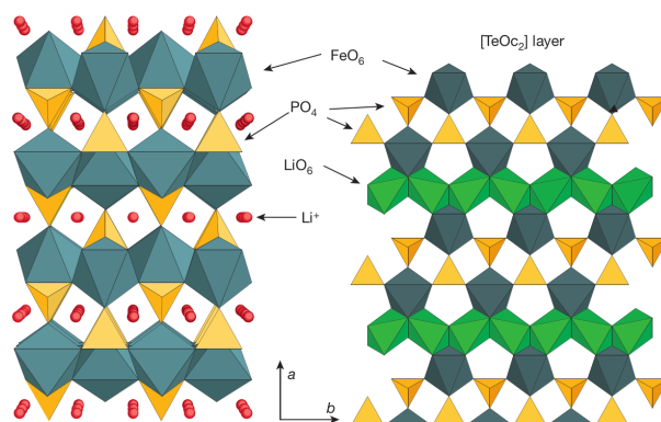
FIGURE 16 – Structure de l'olivine \text{LiFePO}_4 dans la projection le long de [001].
