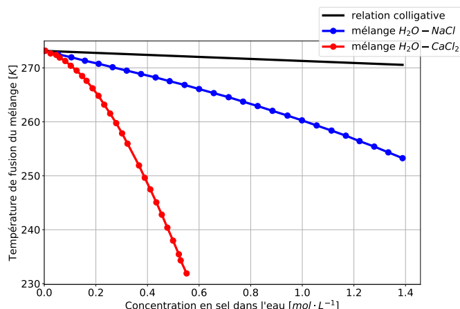
FIGURE 10 – Évolution de température de fusion d'un mélange eau-sel en fonction de la concentration en sel dans le cas NaCl et \text{CaCl}_2 .
