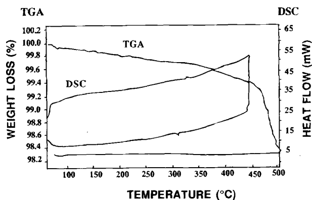
FIGURE 17 – Analyse par thermogravimétrie et par analyse calorimétrique différentielle de la phase délithié FePO 4 en présence d'une atmosphère inerte (diazote).
