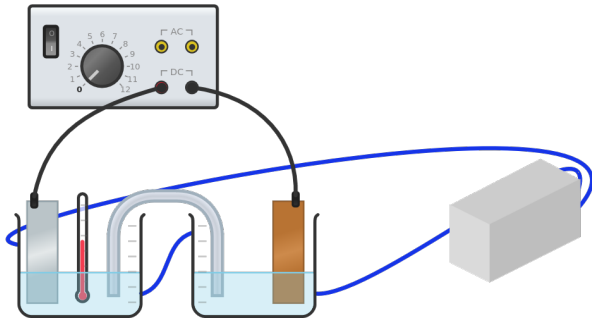
Figure 4 – Montage de base de l'expérience où la pile est branchée à un générateur de tension.
