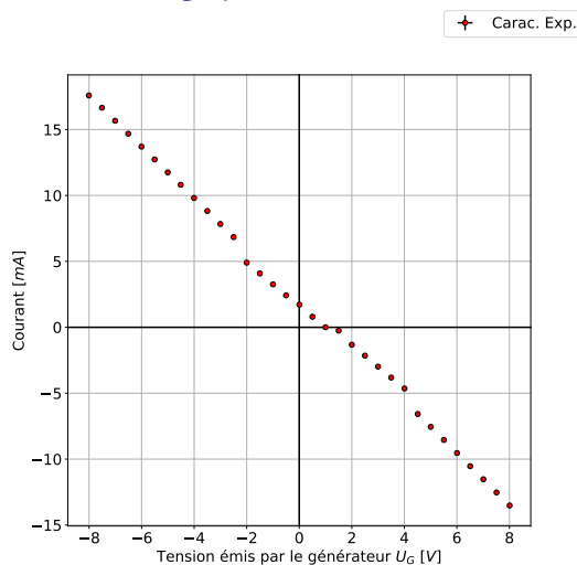
Figure 6 – Caractéristique expérimentale de la pile Daniell à 24.9\text{ }^{\circ}\text{C} .
