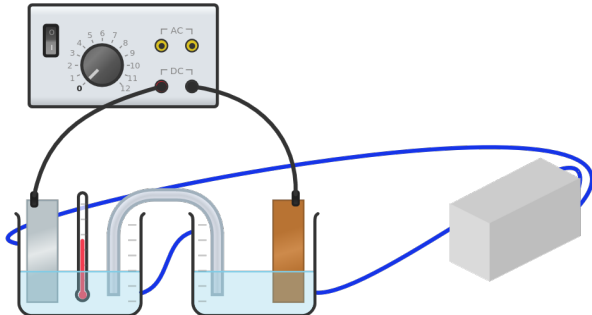
Figure 4 – Montage de base de l'expérience où la pile est branchée à un générateur de tension.
