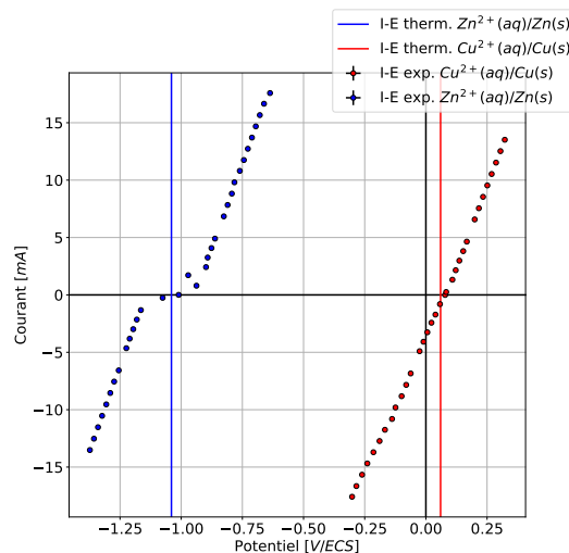
Figure 11 – Courbe courant-potential à une électrode de cuivre et une électrode de zinc.
