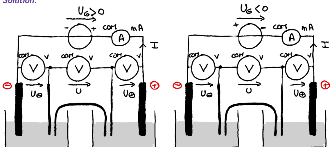
Figure 5 – Le montage à gauche permet la mesure des tensions positives de la pile, le montage de droite des tensions négatives de la pile
