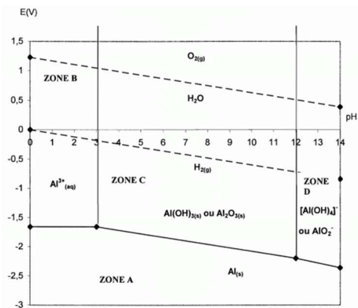
Figure 1 – Diagramme E-pH de l'aluminium et de l'eau à 25 °C [la convention de tracé est fixée à 1 \text{ mol L}^{-1} ]
