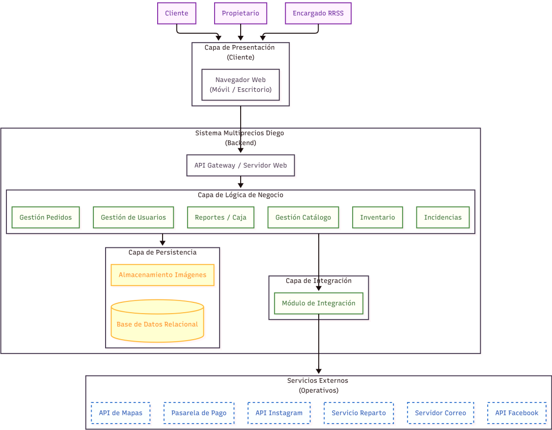
Figura 2: Diagrama de arquitectura del sistema
