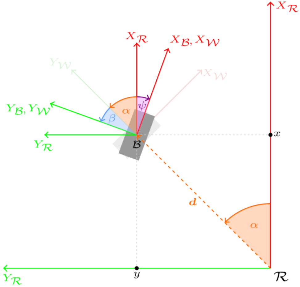
Figura 2: Orientación de la rueda en la dirección de interés, mediante el ángulo \beta .
