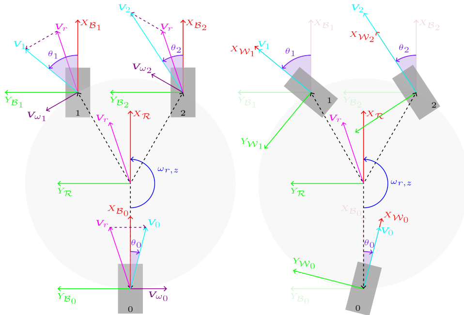
Figura 9: Configuración Y. Izquierda: Cálculo del vector velocidad de cada rueda, V_i . Derecha: Orientación final que cada rueda debe adoptar ( \theta_i ) para alinear su dirección de rodadura con el vector de velocidad V_i .
