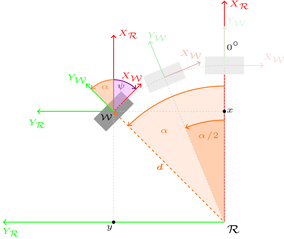
Figura 1: Posicionamiento 2D de una rueda respecto al SC del robot, \mathcal{R} .
