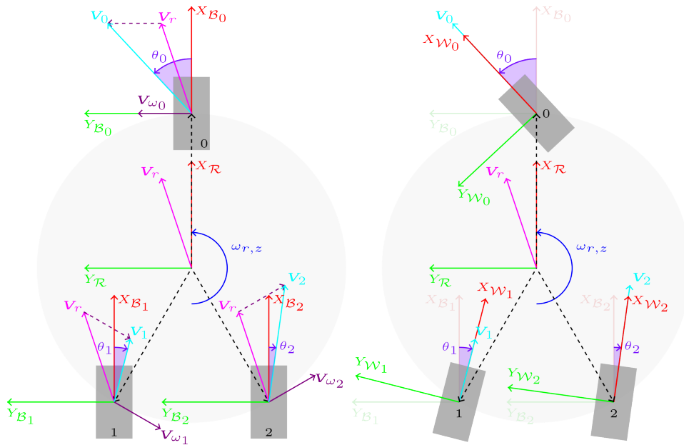
Figura 8: Configuración Y-invertida. Izquierda: Cálculo del vector velocidad de cada rueda, V_i . Derecha: Orientación final que cada rueda debe adoptar ( \theta_i ) para alinear su dirección de rodadura con el vector de velocidad V_i .
