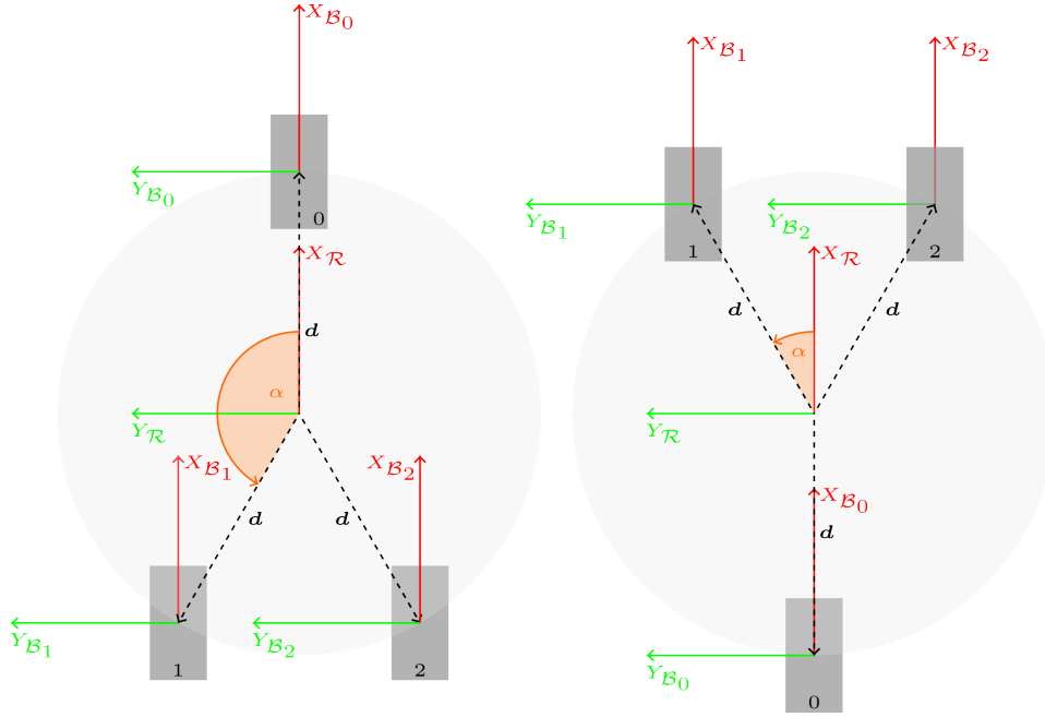
Figura 6: Configuraciones comunes de las ruedas en un sistema three swerve drive (izquierda: configuración Y-invertida, derecha: configuración Y)
