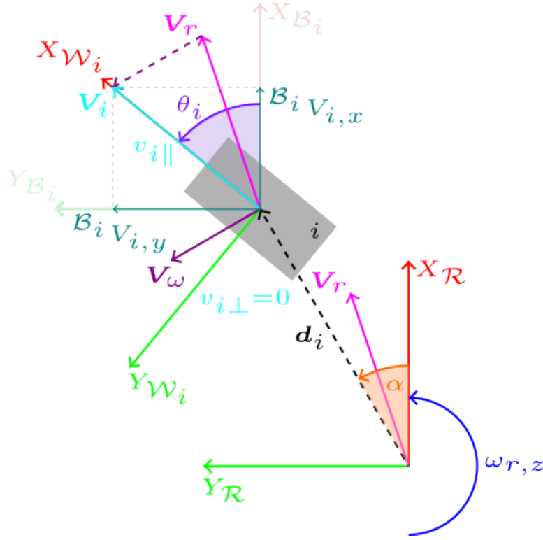
Figura 7: Rueda convencional orientable alineada con su vector de velocidad \mathbf{V}_i mediante una rotación de ángulo \theta_i respecto de su SC base \mathcal{B}_i . La dirección de rodadura queda definida por el eje X_{\mathcal{W}_i} del SC fijo a la rueda i , \mathcal{W}_i .
