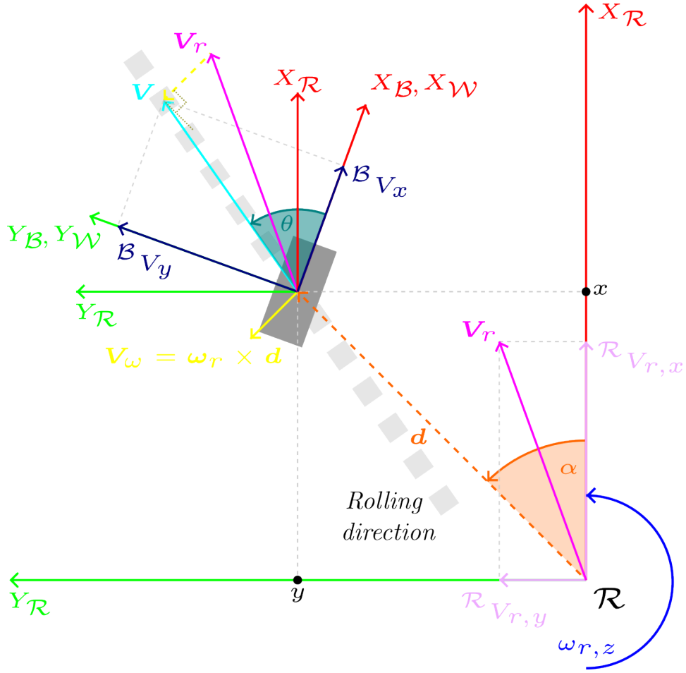
Figura 4: V_r es el vector velocidad del robot. V_\omega es el vector velocidad tangencial de la rueda debido a la rotación del chasis. V es el vector velocidad de la rueda orientable.
