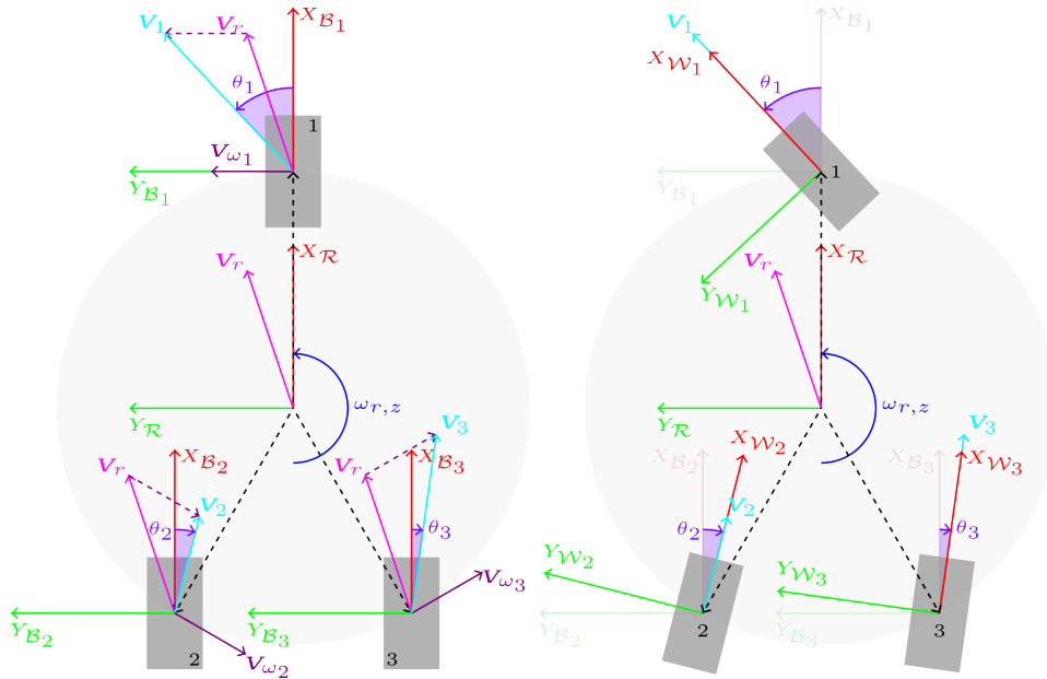
Figura 8: Configuración Y-invertida. Izquierda: Cálculo del vector velocidad de cada rueda, \mathbf{V}_i . Derecha: Orientación final que cada rueda debe adoptar ( \theta_i ) para alinear su dirección de rodadura con el vector de velocidad \mathbf{V}_i .
