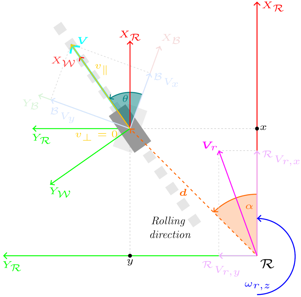
Figura 5: Relación entre las componentes del vector velocidad de la rueda \mathbf{V} en el SC \mathcal{B} , {}^B V_x y {}^B V_y , y en el SC \mathcal{W} , v_{\parallel} y v_{\perp} .
