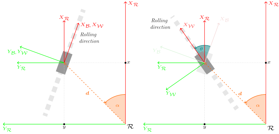
Figura 3: Izquierda: Rueda convencional no orientable, con direcci3n de rodadura fija. Derecha: Rueda convencional orientable, con direcci3n de rodadura variable, que se consigue pivotando la rueda un 3ngulo \theta respecto del SC base de la rueda, \mathcal{B} .
