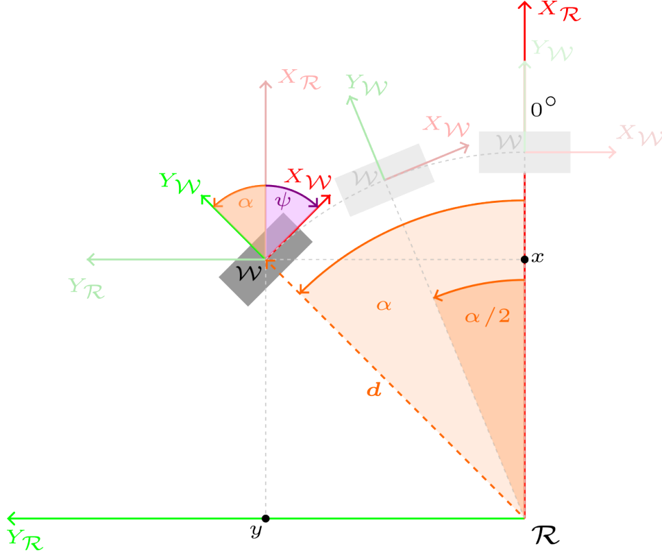
Figura 1: Posicionamiento 2D de una rueda respecto al SC del robot, \mathcal{R} .
