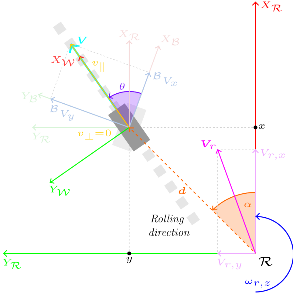
Figura 5: Relación entre el vector velocidad de la rueda en el SC \mathcal{B} , {}^{\mathcal{B}}\mathbf{V} y en el SC \mathcal{W} , {}^{\mathcal{W}}\mathbf{V} para una rueda convencional orientable.
