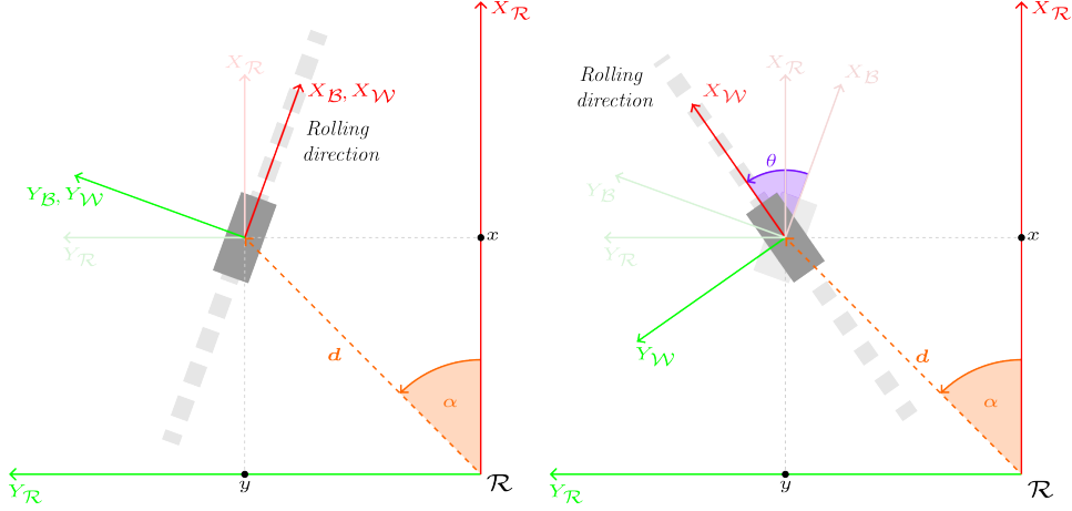
Figura 3: Izquierda: Rueda convencional no orientable. El SC \mathcal{W} , fijo a la rueda, coincide todo el tiempo con el SC base de la rueda, \mathcal{B} . La dirección de rodadura está indicada por la dirección del eje X_W y en este caso es fija. Derecha: Rueda convencional orientable. El SC \mathcal{W} , fijo a la rueda, va cambiando su orientación ( \theta ) respecto del SC base de la rueda, \mathcal{B} . La dirección de rodadura está indicada por la dirección del eje X_W y puede variar a lo largo del tiempo.
