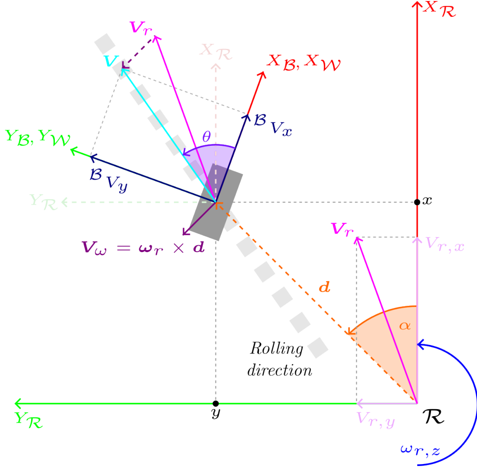
Figura 4: \mathbf{V}_r es el vector velocidad lineal del robot expresado en el SC \mathcal{R} . \mathbf{V}_\omega es el vector velocidad tangencial de la rueda debido a la rotación del chasis. \mathbf{V} es el vector velocidad lineal de la rueda.
