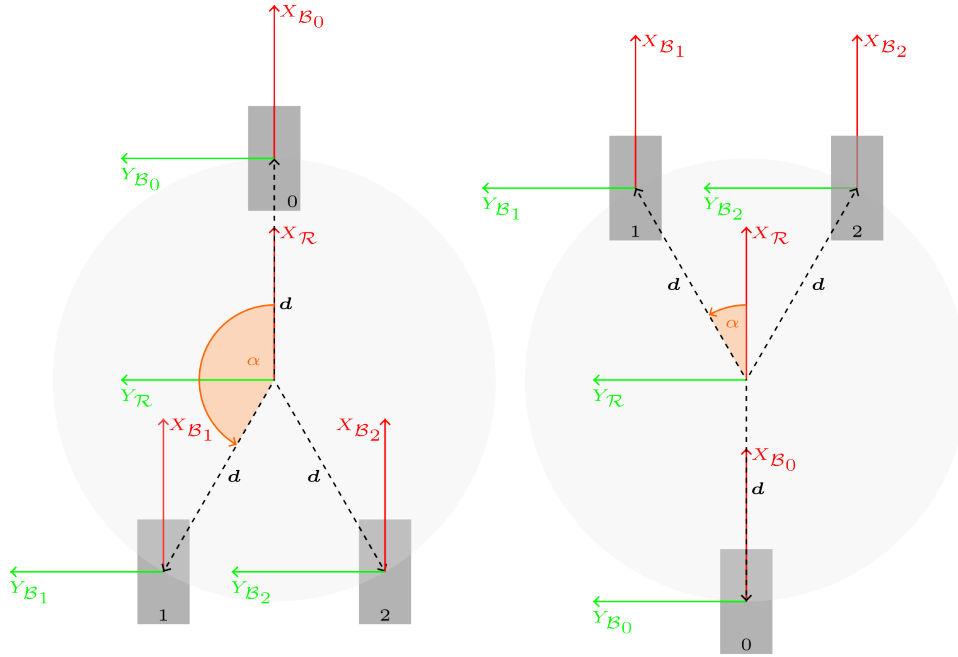
Figura 6: Disposiciones de las 3 ruedas activas en un robot. Izquierda: Configuración Y-invertida. Derecha: configuración Y)
