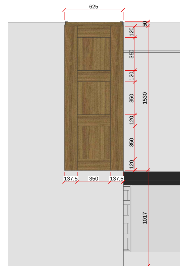
PAINEL COM NICHOS - ESC. 1:25
