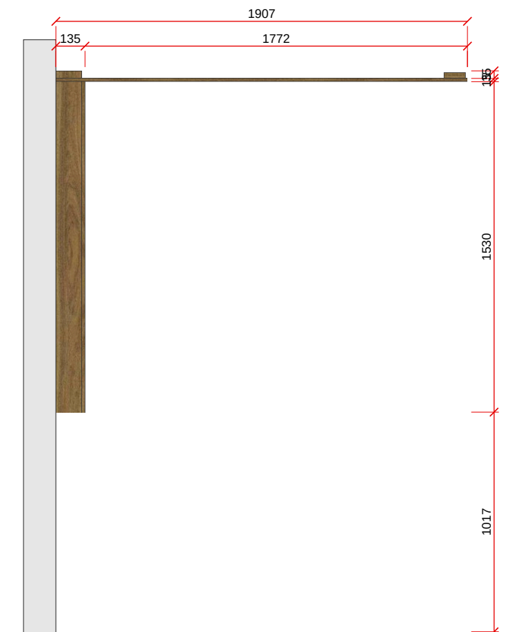
PAINEL COM NICHOS - LATERAL - ESC. 1:25
