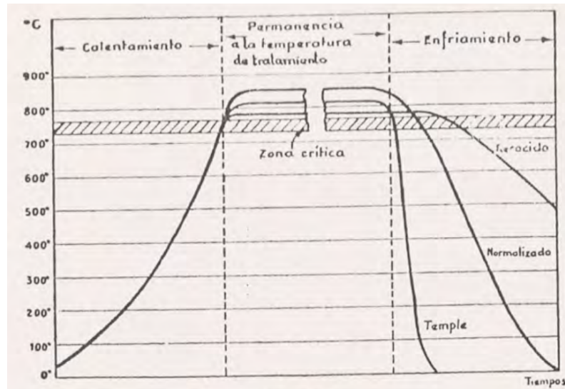
Figura 1: Como la velocidad de enfriamiento afecta al tratamiento termico.
