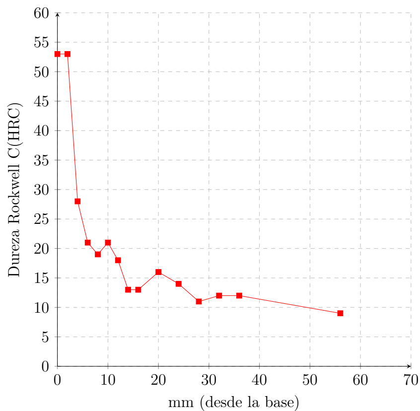
Figura 7: Evolucion de la dureza segun la distancia.
