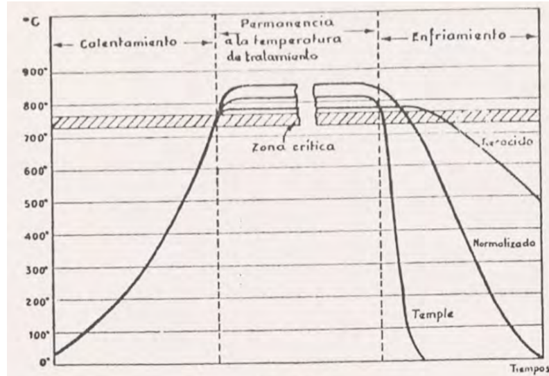
Figura 1: Como la velocidad de enfriamiento afecta al tratamiento termico.
