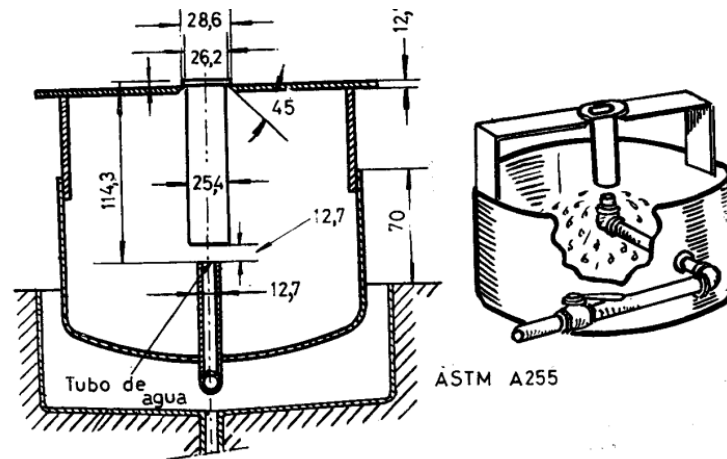
Figura 2: esquema de montaje y probeta para el ensayo Jominy.
