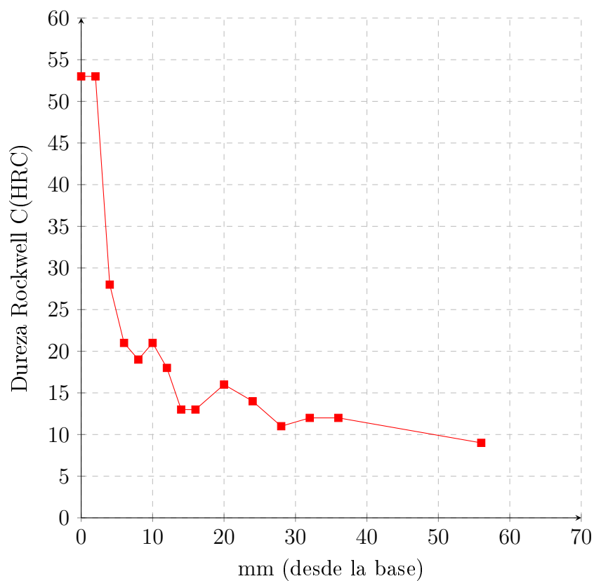
Figura 5: Evolucion de la dureza segun la distancia.
