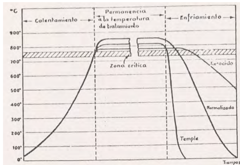
Figura 3: Como la velocidad de enfriamiento afecta al tratamiento termico.
