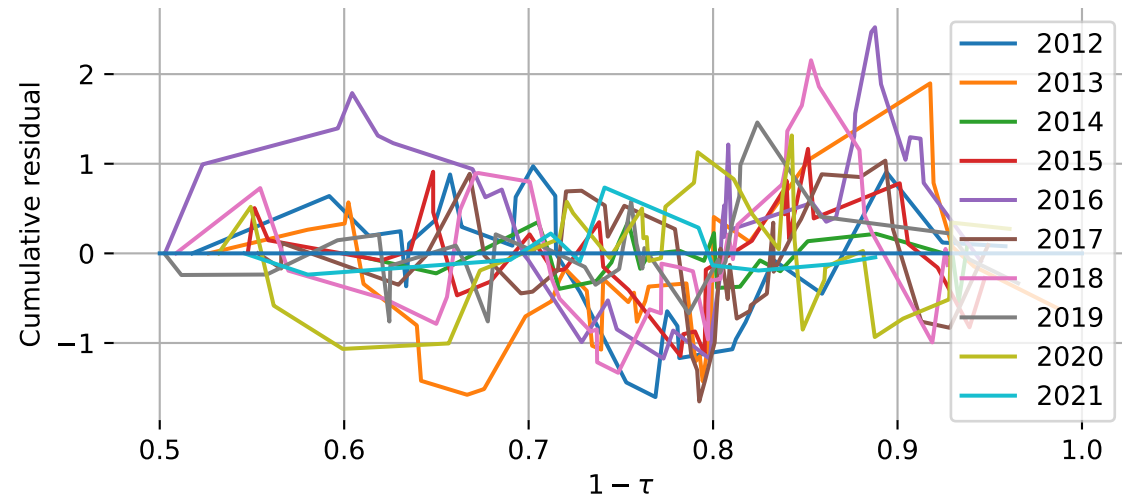
Quadratic
