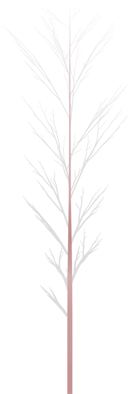
A. rubrum 2
