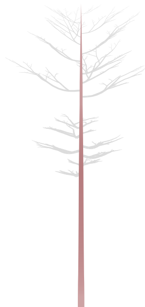
N. sylvatica
