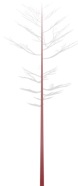
N. sylvatica
