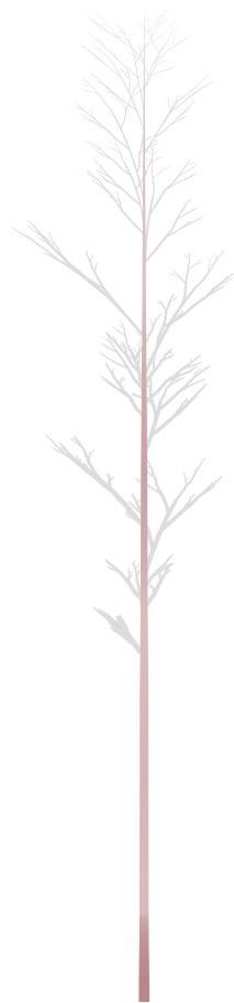
Q. rubra
