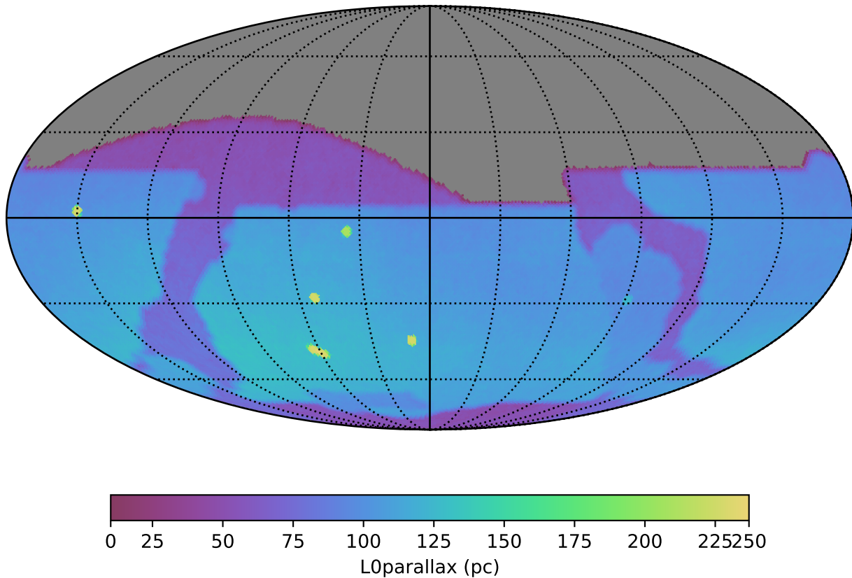
baseline_v5.0.0_10yrs : L0parallax
