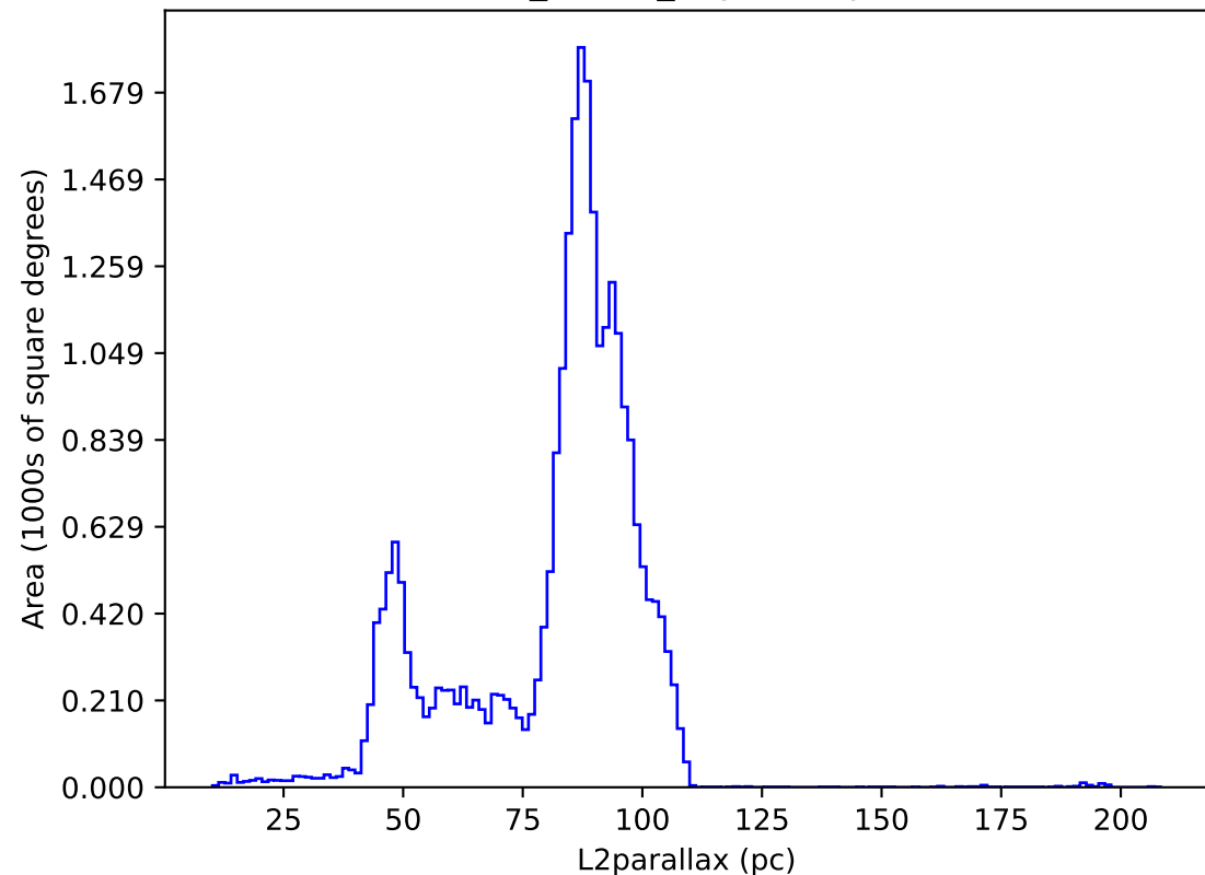
baseline_v5.0.0_10yrs : L2parallax
