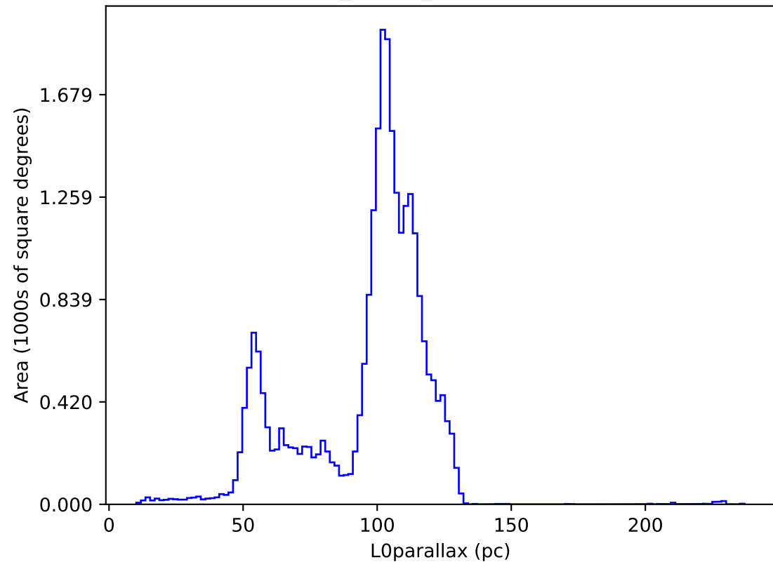
baseline_v5.0.0_10yrs : L0parallax
