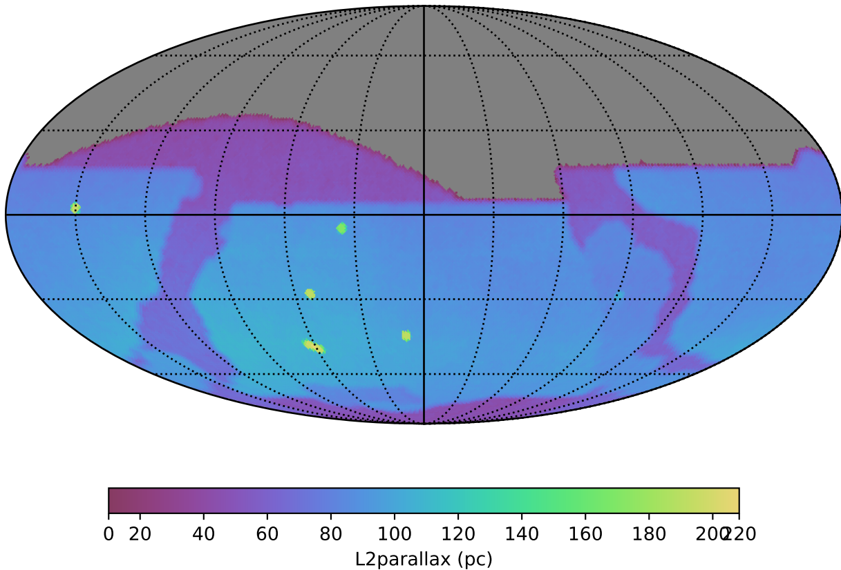
baseline_v5.0.0_10yrs : L2parallax
