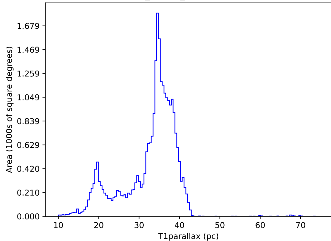
baseline_v5.0.0_10yrs : T1parallax
