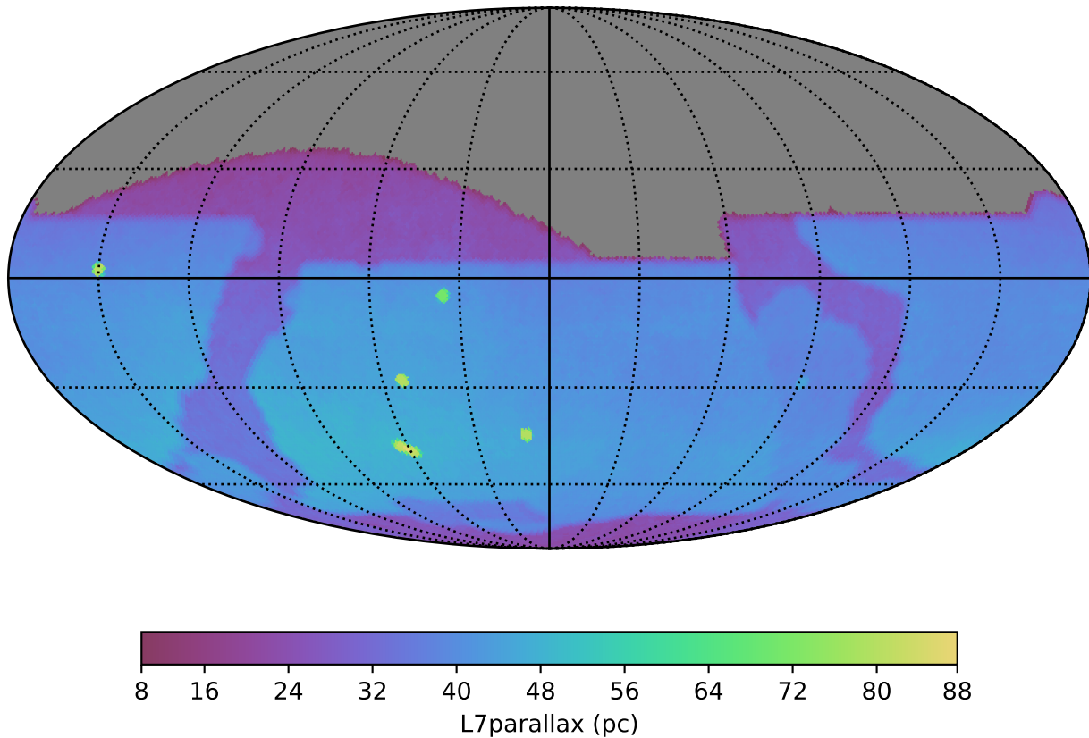
baseline_v5.0.0_10yrs : L7parallax
