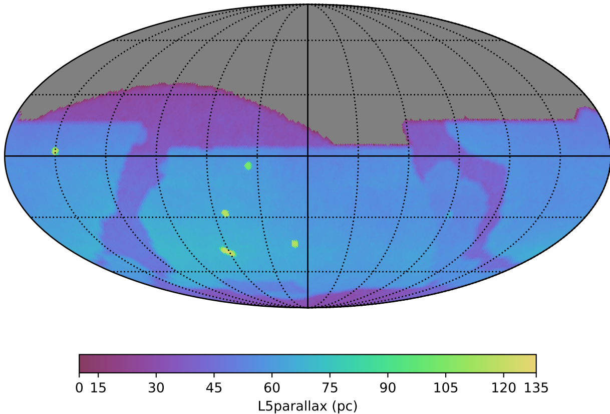
baseline_v5.0.0_10yrs : L5parallax
