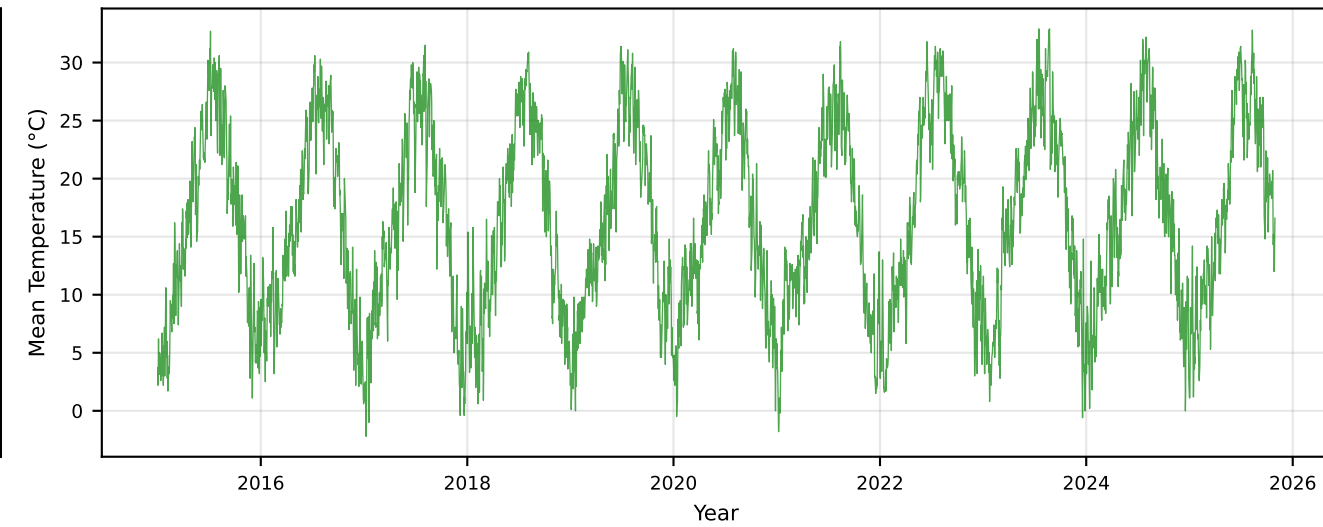
LLEIDA (003942) Elev: 186m
