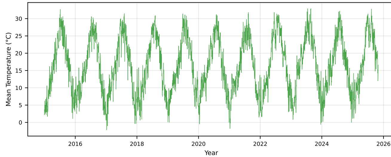
LLEIDA OBSERVATORIO (003943) Elev: 199m
