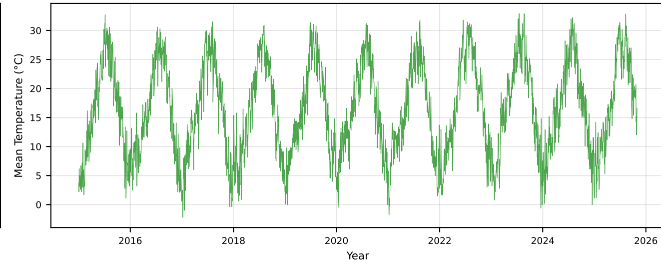
LLEIDA-ESCORNADOR (010905) Elev: 162m
