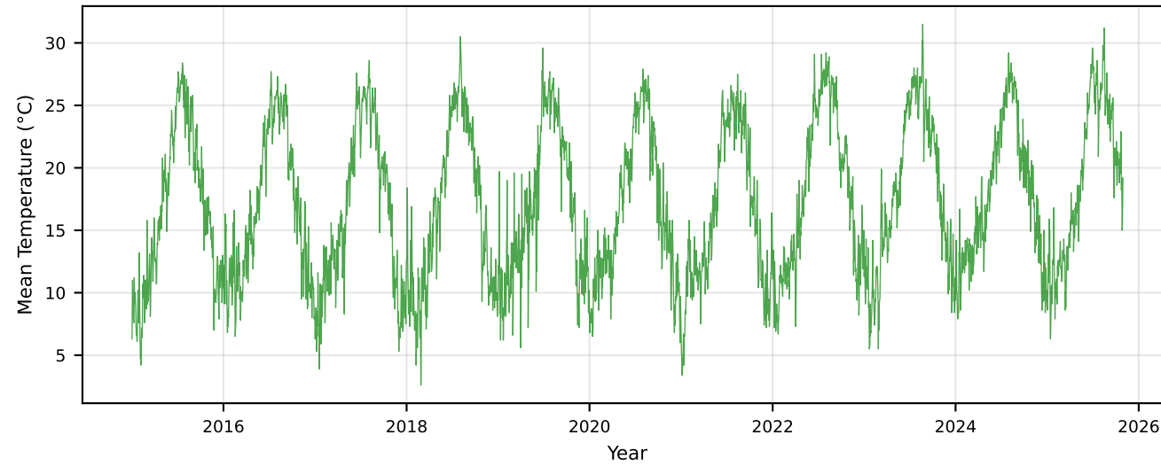
BARCELONA FABRA (000335) Elev: 408m
