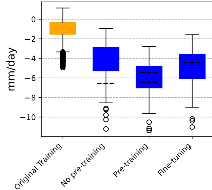
Bias SDII
