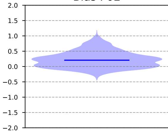
Bias P02
