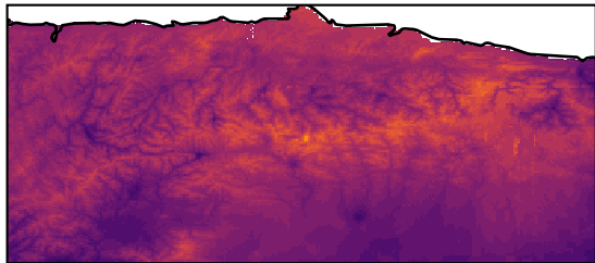
TXx
