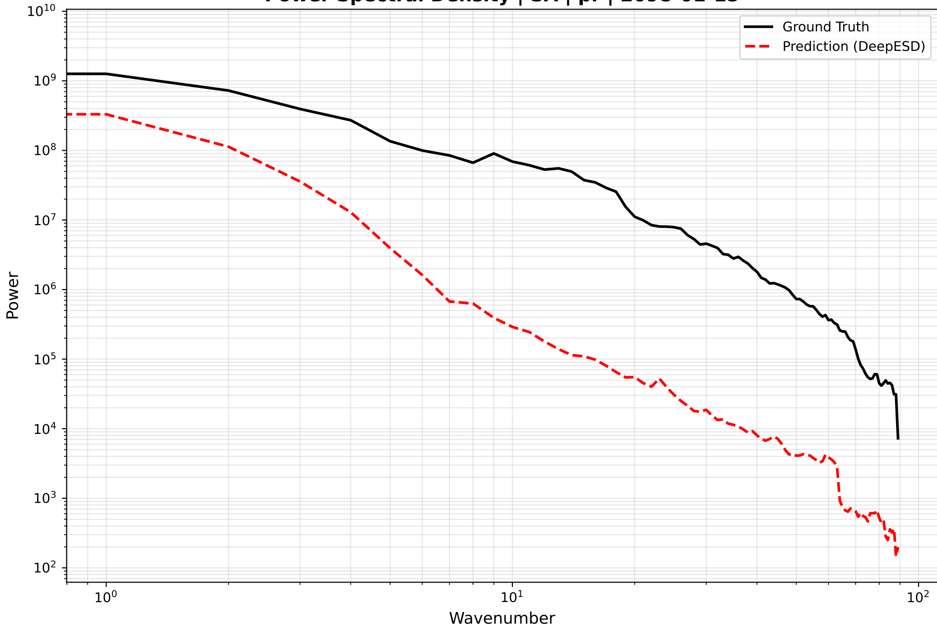
Power Spectral Density | SA | pr | 2098-01-15
