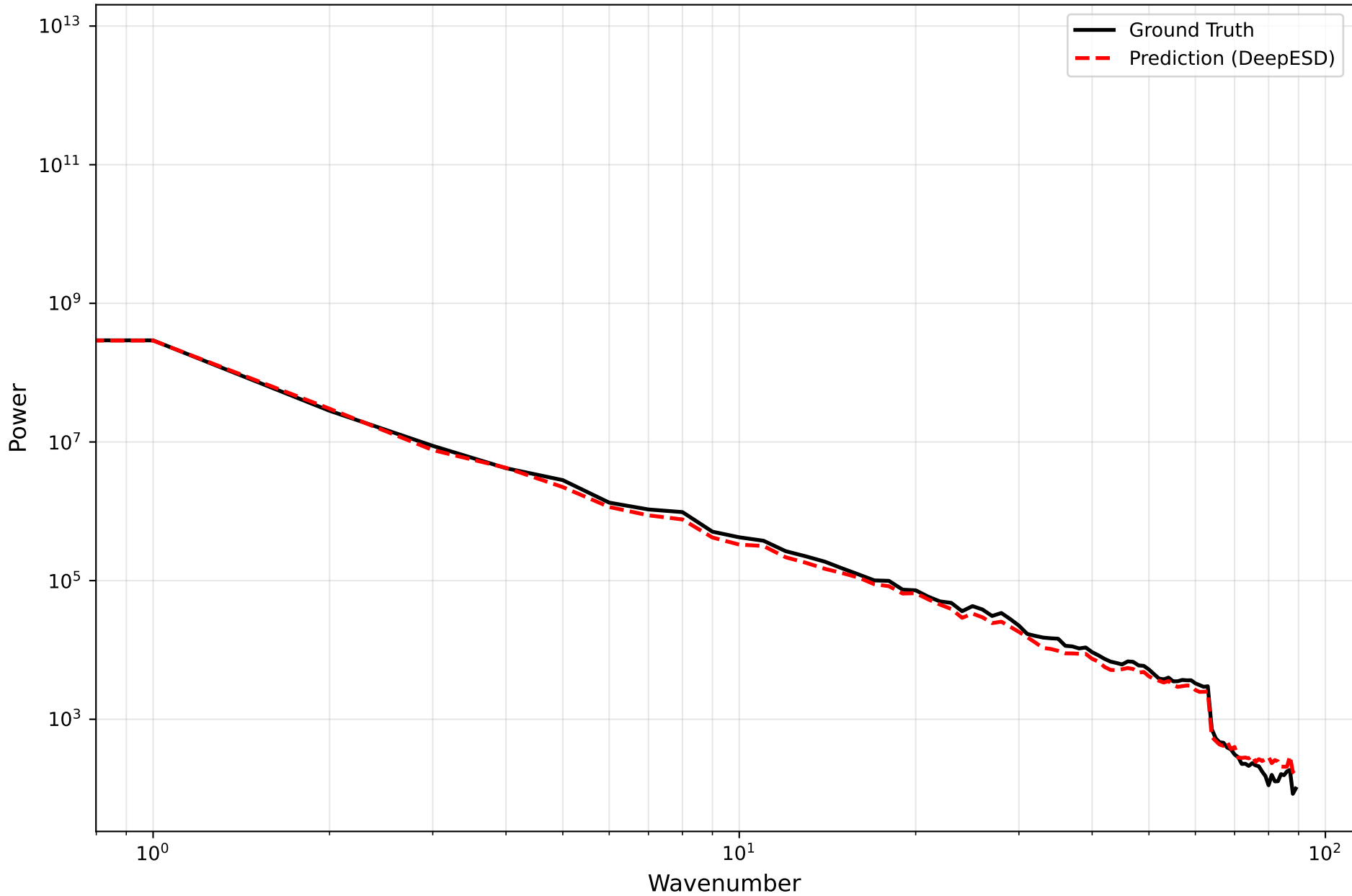
Power Spectral Density | SA | tasmax | 2098-07-15
