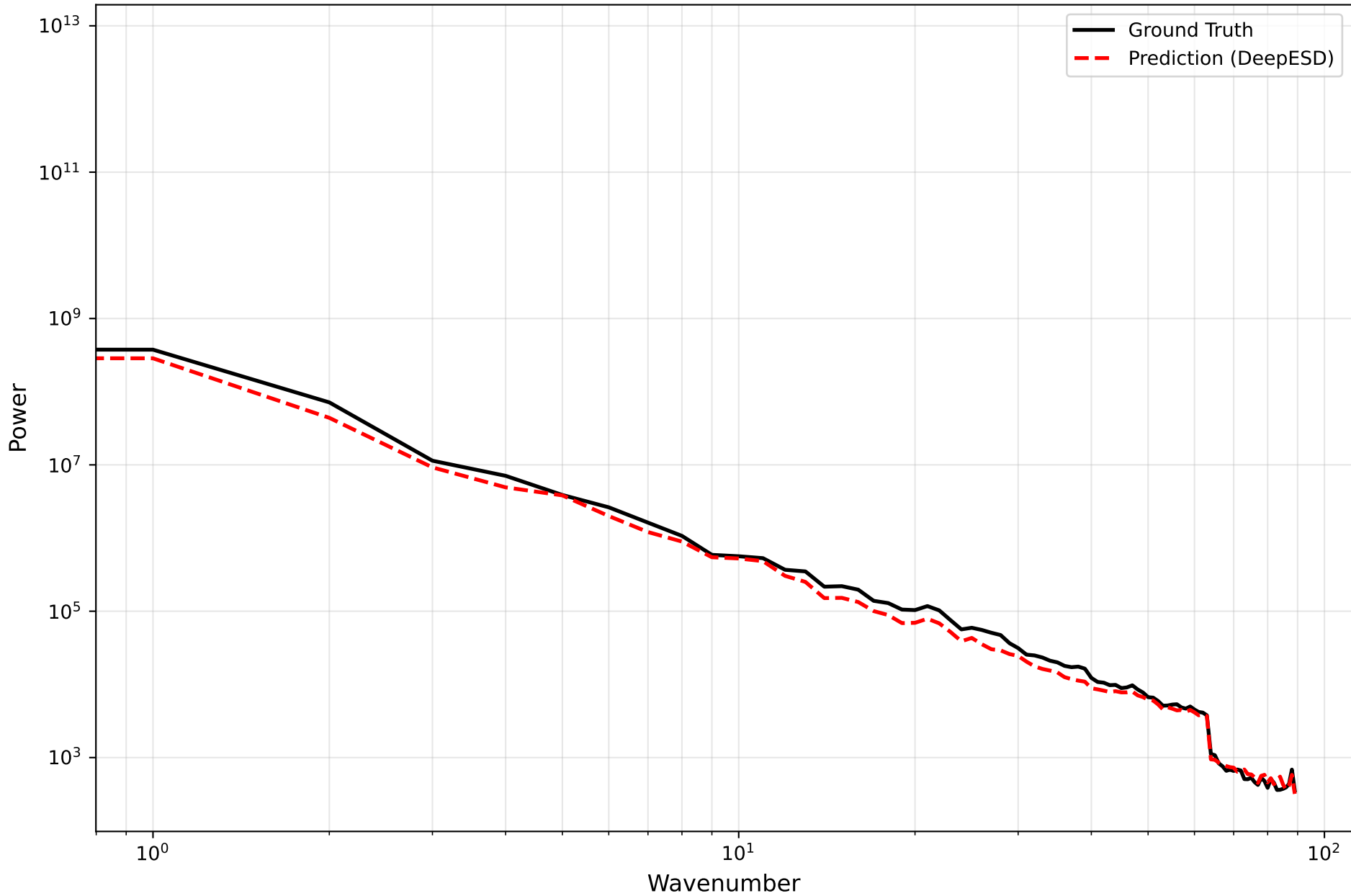
Power Spectral Density | SA | tasmax | 1980-01-15
