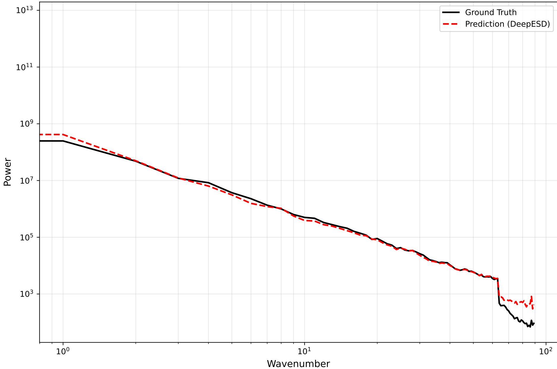
Power Spectral Density | SA | tasmax | 1980-07-15
