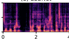
(d) EaBNet
