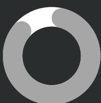
Codeigniter
