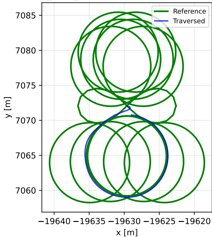
H9_slow_tight: trajectory (lemniscate)
