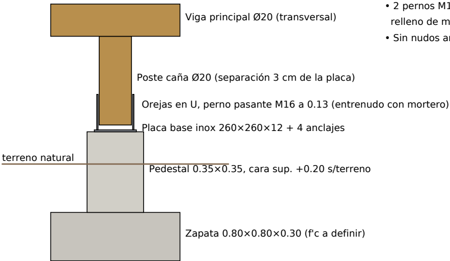
DETALLE 1 — APOYO TIPO (esquemático, sin escala exacta)
