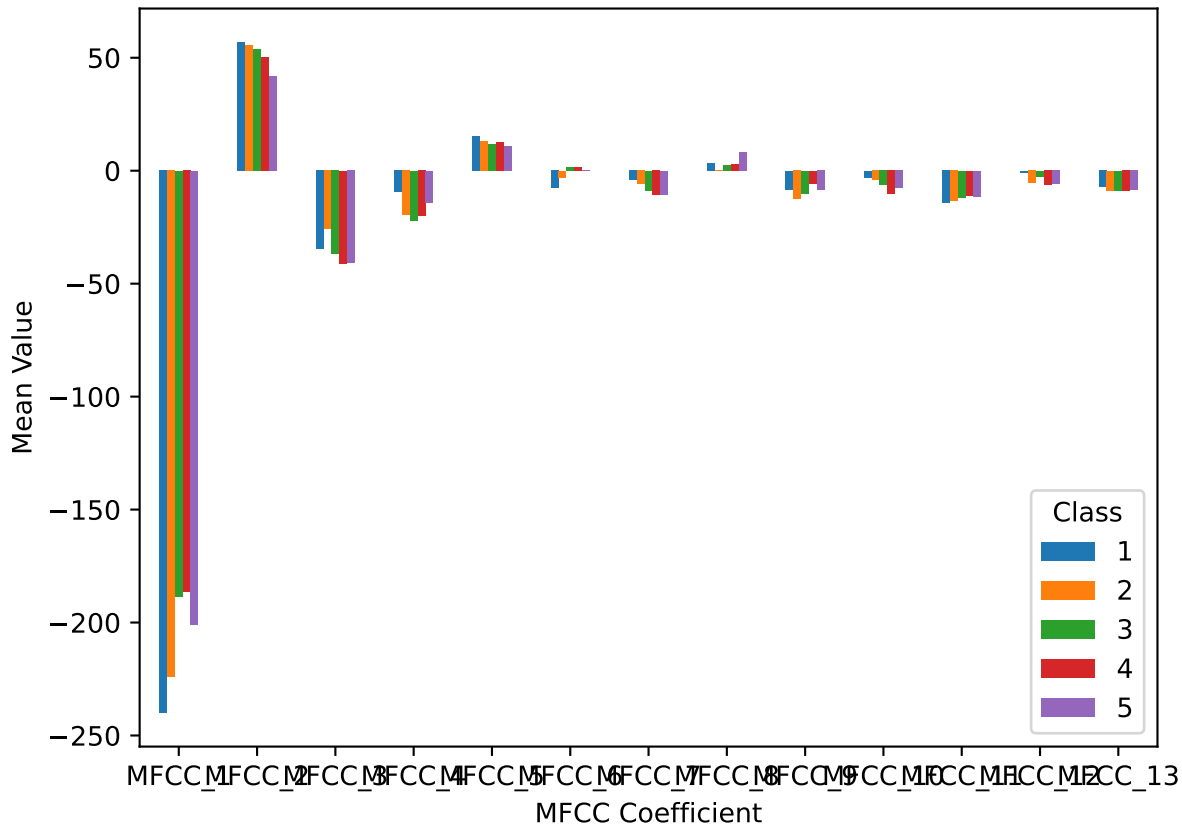
Mean MFCC Values per Class
