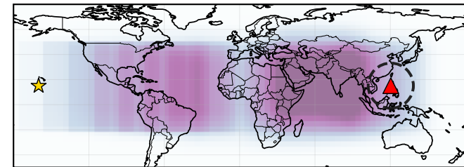
D. \text{SO}_2
