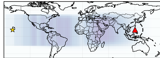
E. \text{SO}_4
