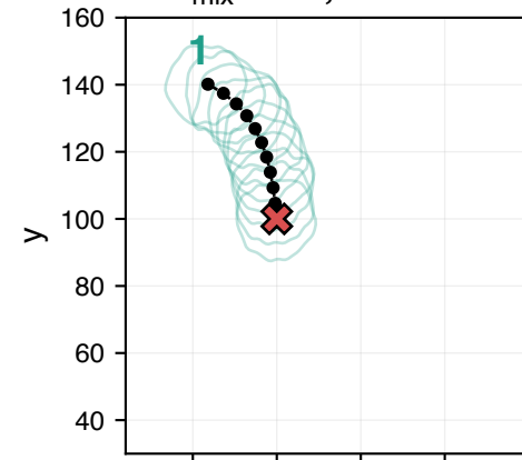
L. \alpha_{\text{mix}} = 0.8 , Var. 1
