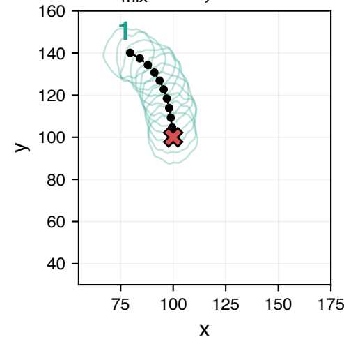
L. \alpha_{\text{mix}} = 0.8 , Var. 1
