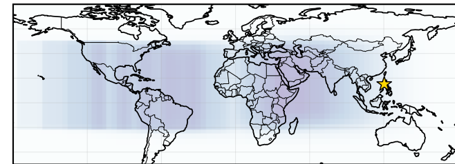
E. \text{SO}_4
