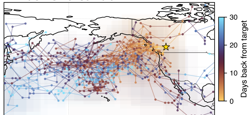
A. TraCE-ST ensemble
