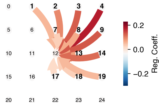
B. Elastic-Net: Var. 1_{t-1} \rightarrow \text{Var. } 1_t
