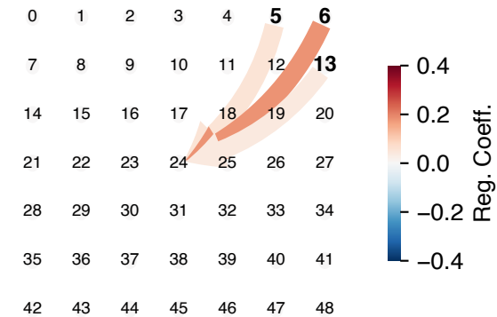
D. DYNOTEARS: Var. 2_{t-1} \rightarrow \text{Var. } 1_t
