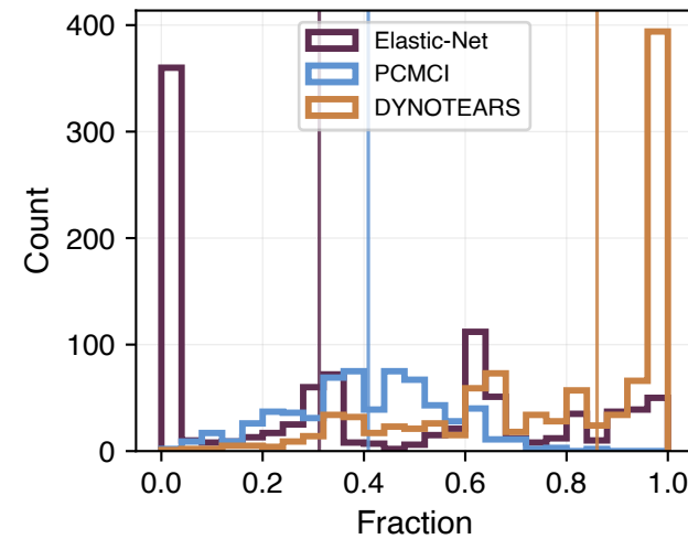
G. Mean Var. 2 fraction
