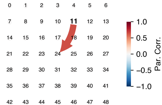
C. PCMCi: Var. 1_{t-1} \rightarrow \text{Var. } 1_t
