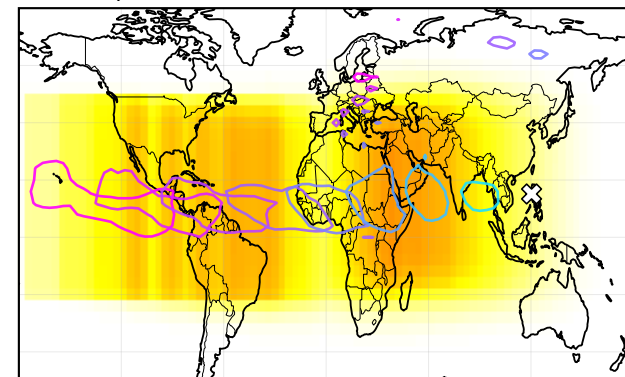
K. \text{SO}_4
