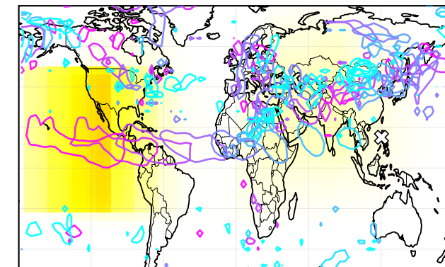
M. AOD
