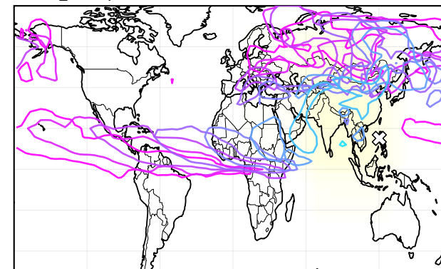
L. \text{H}_2\text{SO}_4
