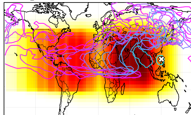
J. \text{SO}_2
