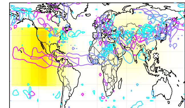
M. AOD
