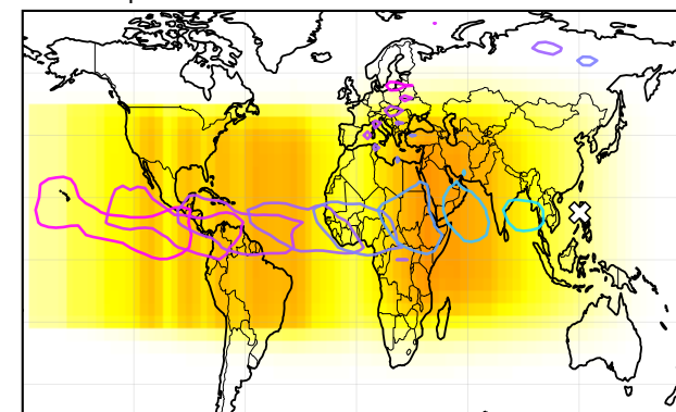
K. SO_4
