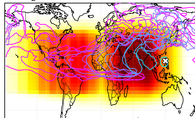
J. SO_2
