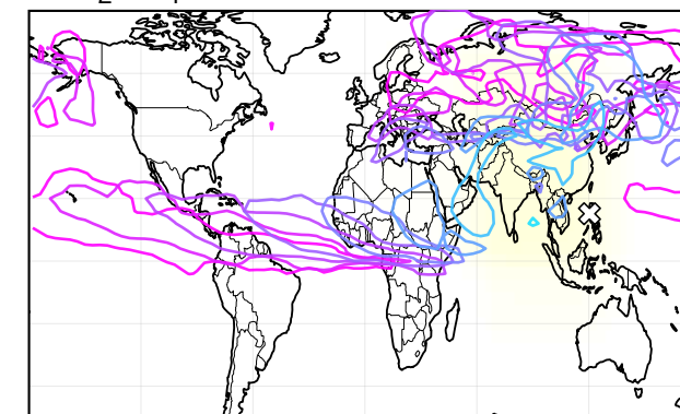
L. H_2SO_4
