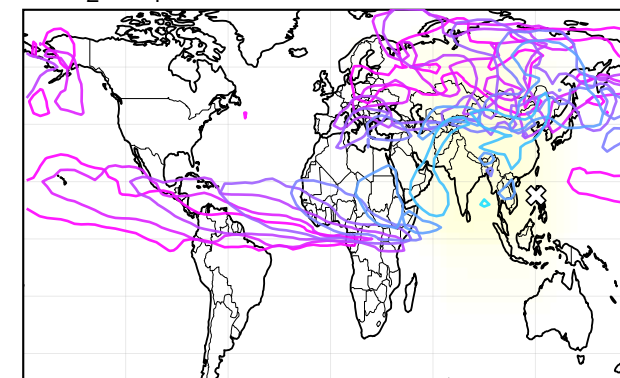
L. \text{H}_2\text{SO}_4
