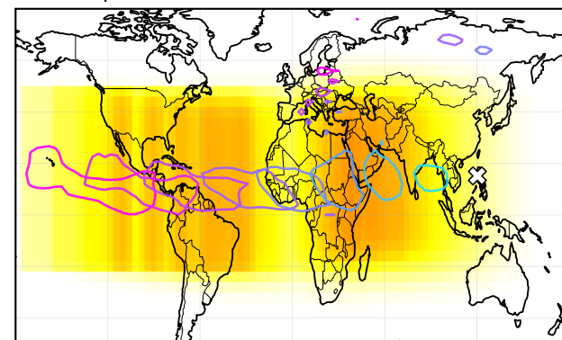
K. \text{SO}_4
