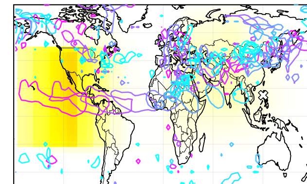
M. AOD
