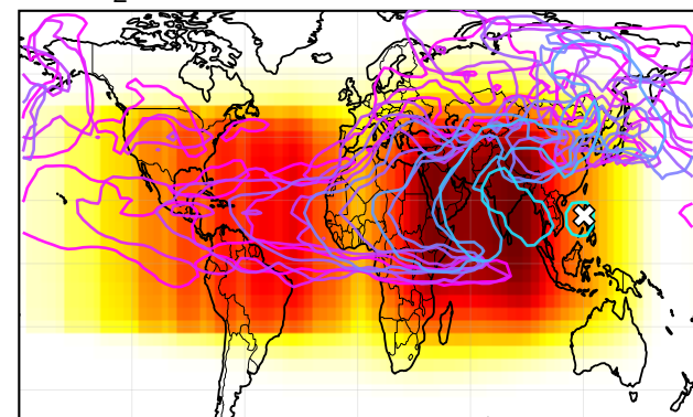
J. \text{SO}_2
