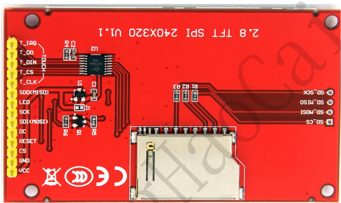
引脚丝印图
